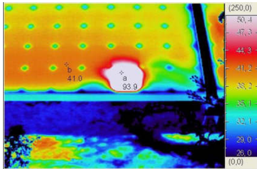
Termografía de un panel fotovoltaico.
