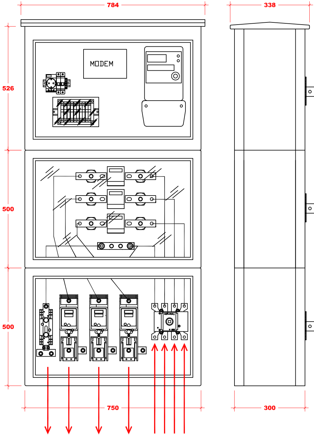
DETALLE APM CPMT-300E-IF C/SECCIONADOR
