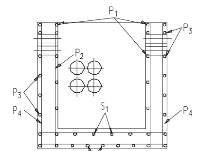
SECCION B-B
