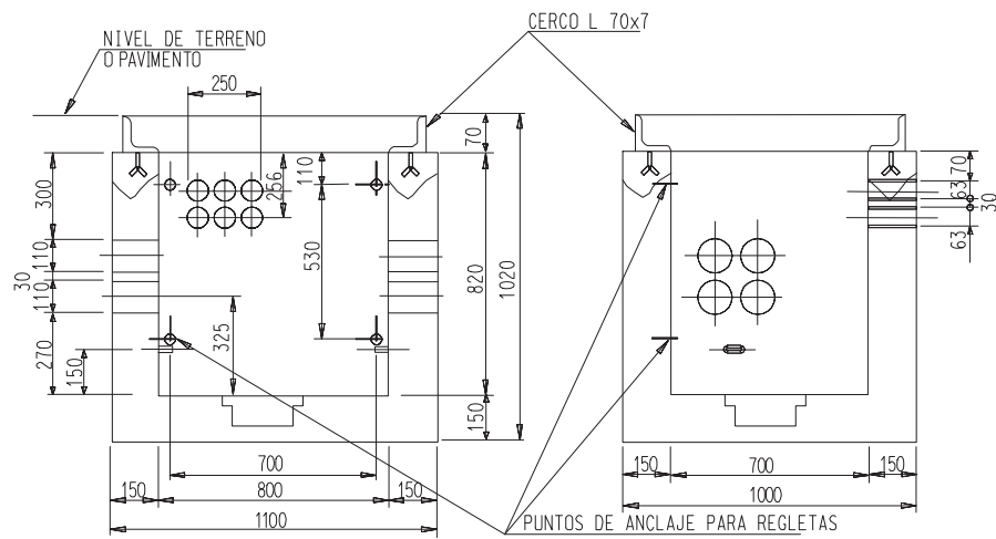
SECCION A-A
