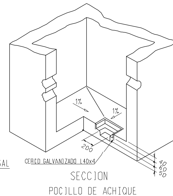
SECCION B-B
