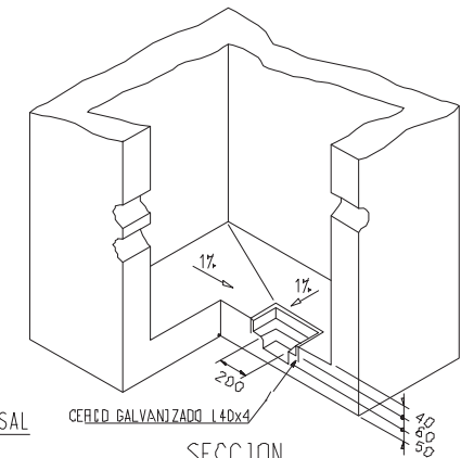
SECCION B-B
