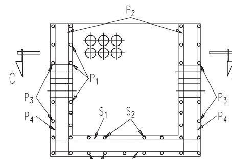
SECCION A-A
