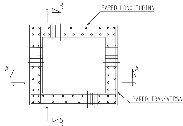
SECCION C-C
