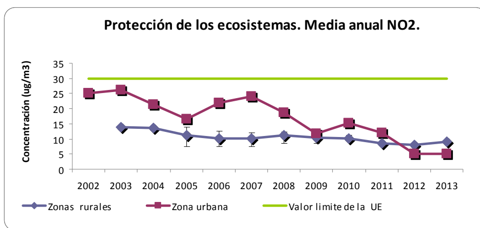
Gráfico 7.- Media anual NO 2 .- Protección de los ecosistemas.
