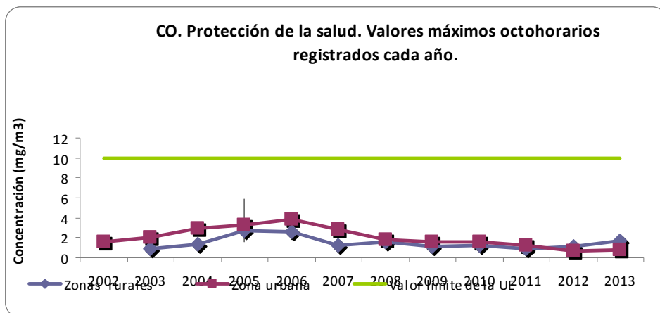
Gráfico 13.- Máximo octohorario de CO.
