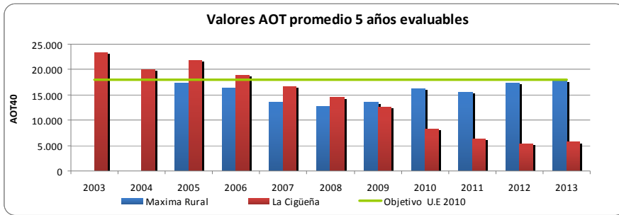
Gráfico 18.- Valor AOT40 de O 3 promedio de 5 años. Protección de los ecosistemas.
