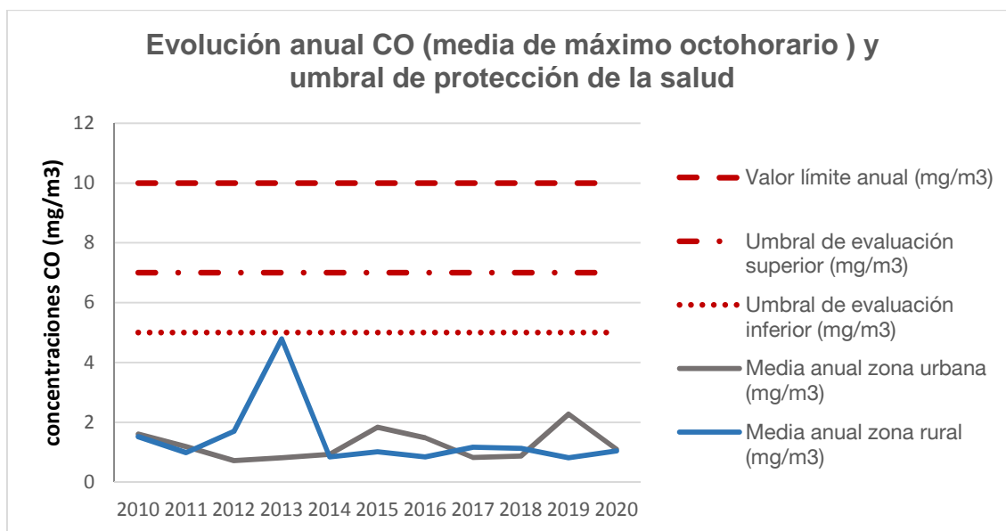
Figura 19. Evolución anual CO para la protección de la salud
