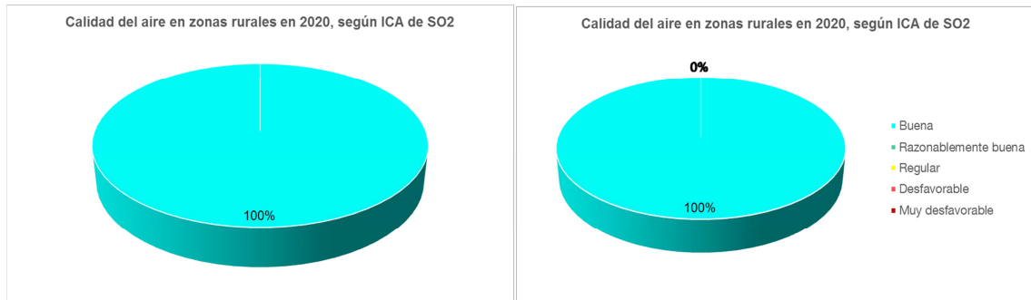
Figura 7. Índice Nacional de Calidad de Aire para SO 2 en 2020
