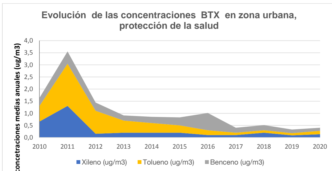
Figura 21. Evolución anual BTX para la protección de la salud en zona urbana
