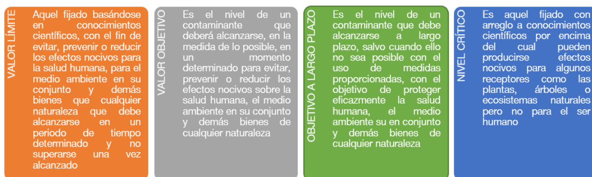
Figura 6. Esquema de los objetivos de calidad y sus definiciones
