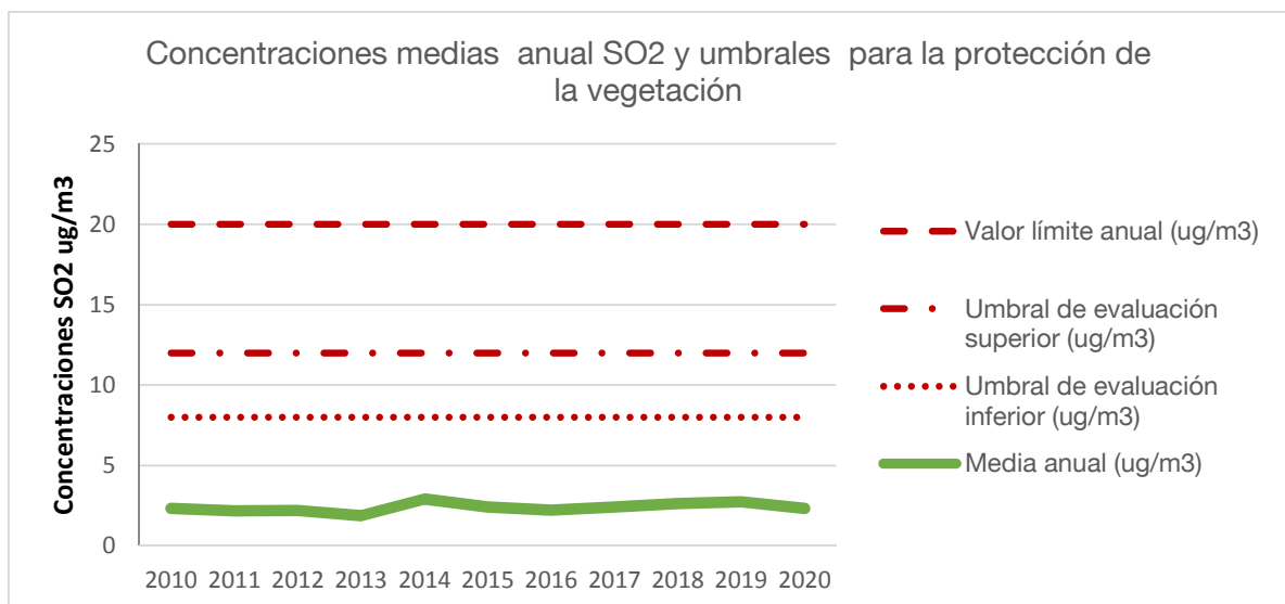
Figura 8. Evolución anual SO 2 para la protección de la vegetación
