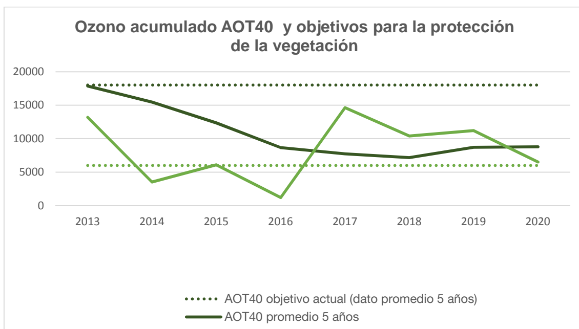
Figura 18. Evolución O_3 para la protección de la vegetación
