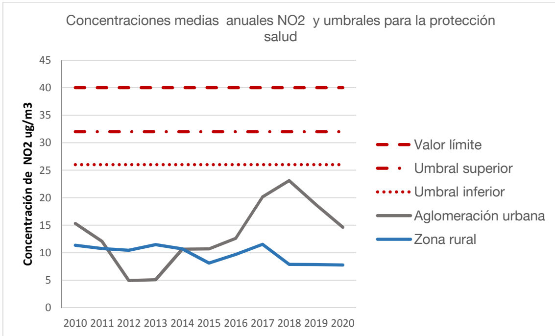
Figura 9. Evolución anual del NO 2 para la protección de la salud
