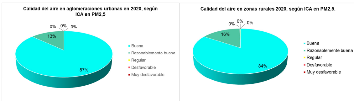
Figura 15. Índice Nacional de Calidad de Aire para PM 2,5 en 2020
