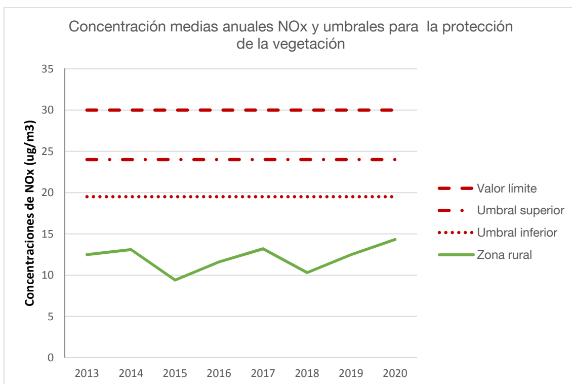
Figura 11. Evolución anual NOx para la protección de la vegetación
