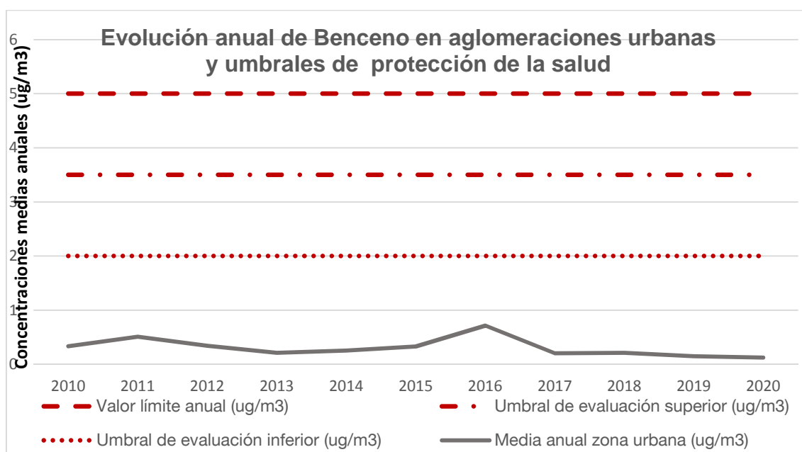
Figura 20. Evolución anual \text{C}_6\text{H}_6 para la protección de la salud en zona urbana
