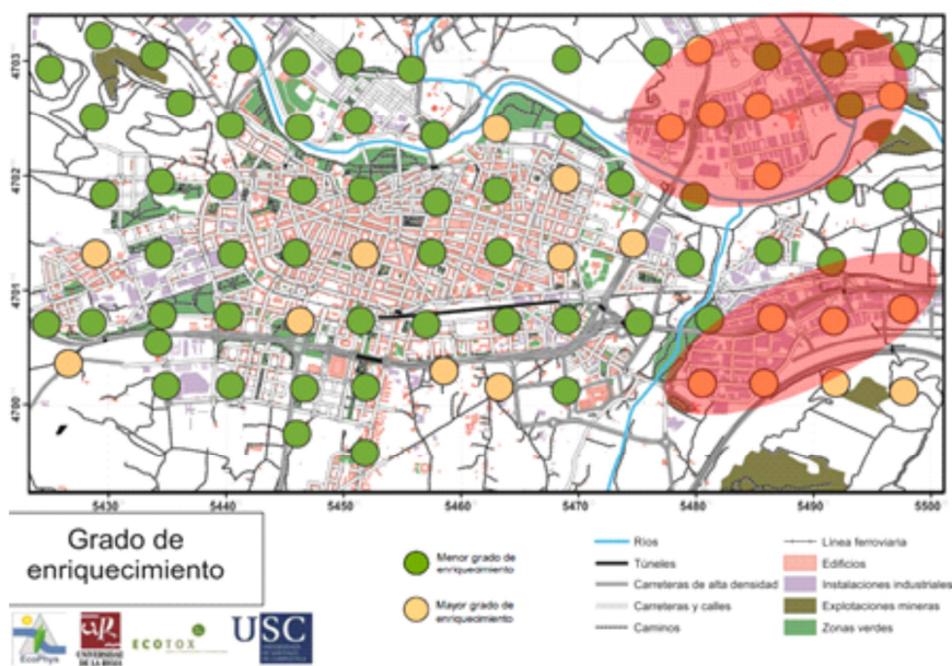
Figura 5. Grado de enriquecimiento en contaminantes en dispositivos Mossphere
