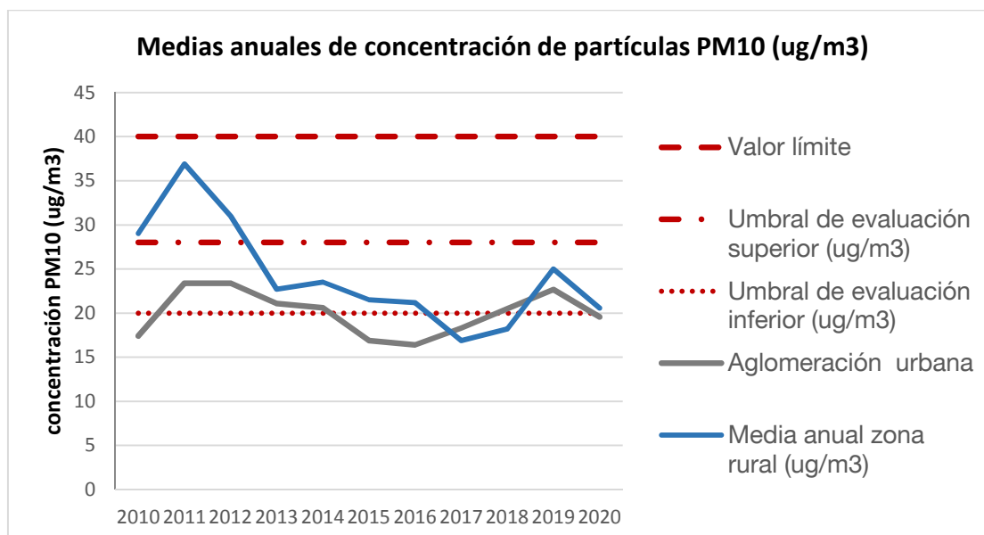
Figura 12. Evolución anual \text{PM}_{10} para la protección de la salud
