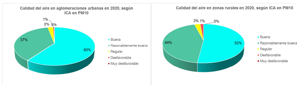
Figura 13. Índice Nacional de Calidad de Aire para PM 10 en 2020
