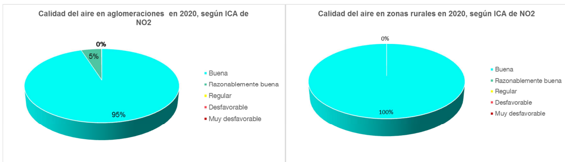
Figura 10. Índice Nacional de Calidad de Aire para NO 2 en 2020
