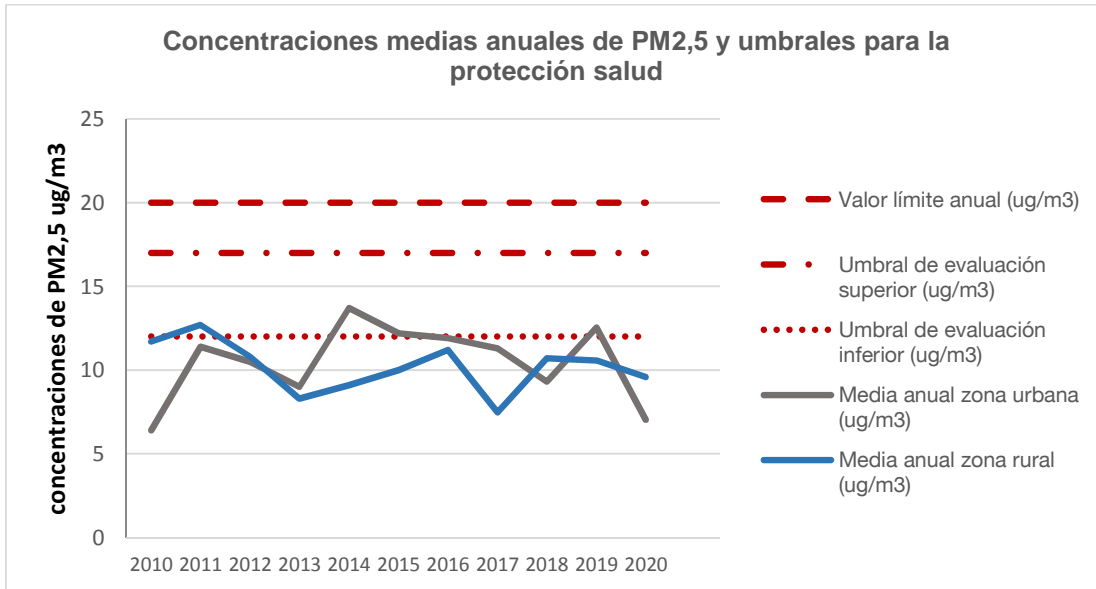
Figura 14. Evolución anual PM 2,5 para la protección de la salud
