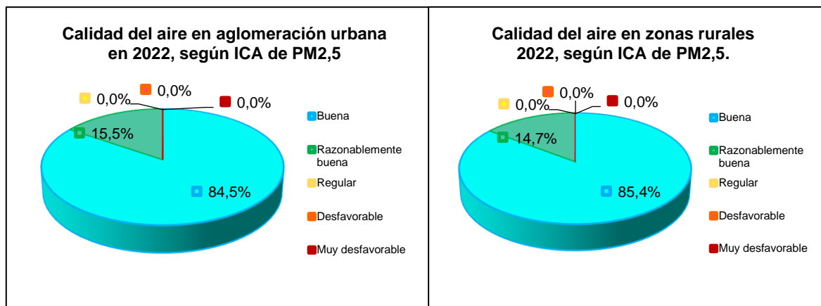
Figura 21. Índice Nacional de Calidad de Aire para PM 2,5 en 2022
