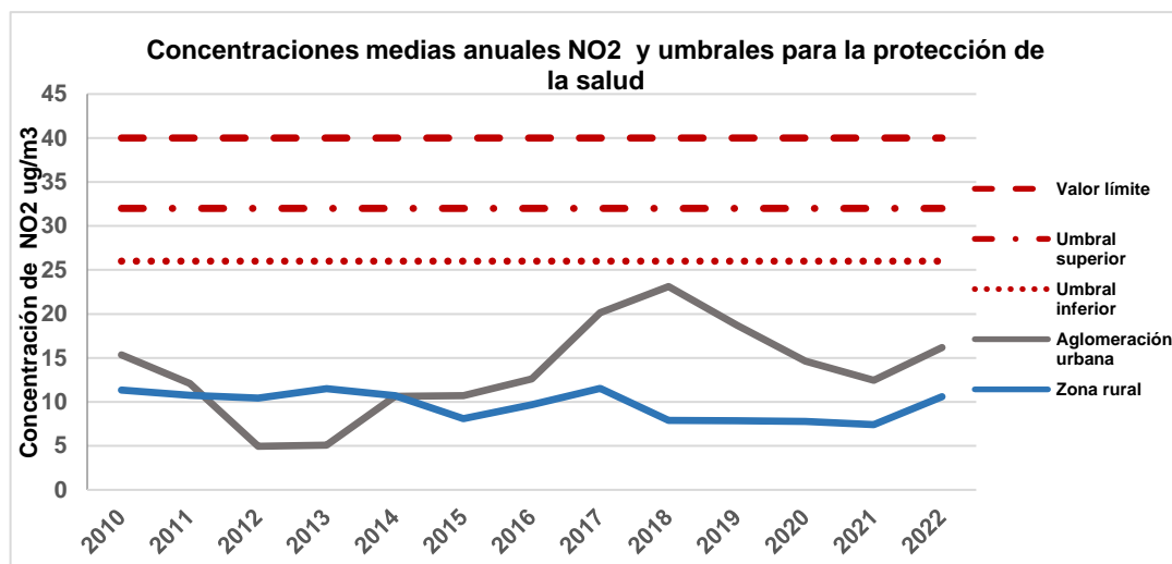
Figura 15. Evolución anual del \text{NO}_2 para la protección de la salud
