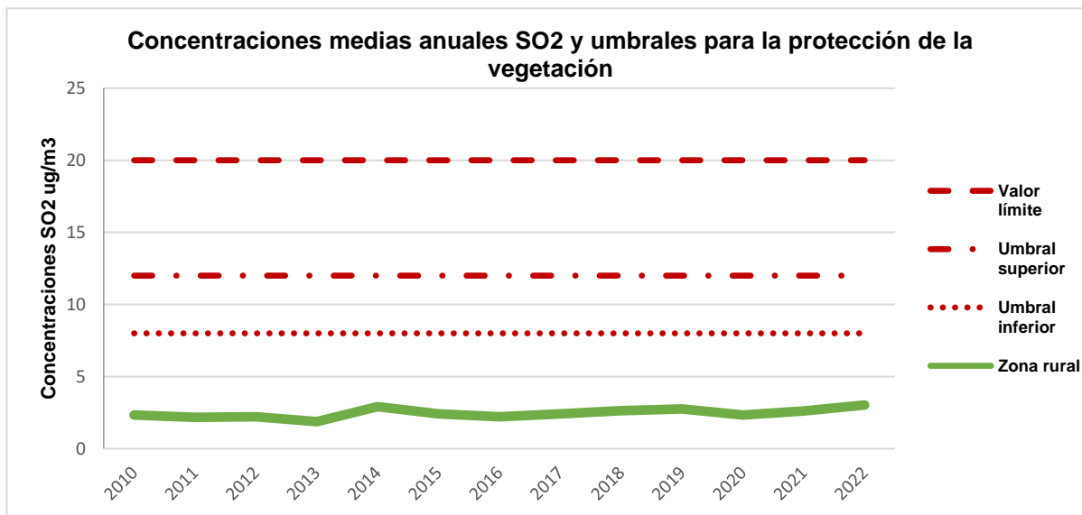
Figura 14. Evolución anual SO 2 para la protección de la vegetación
