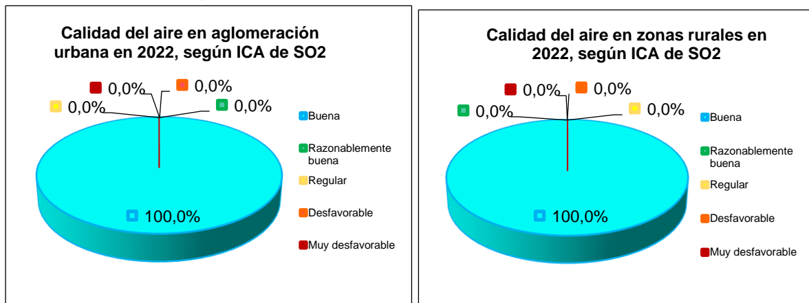
Figura 13. Índice Nacional de Calidad de Aire para SO 2 en 2022
