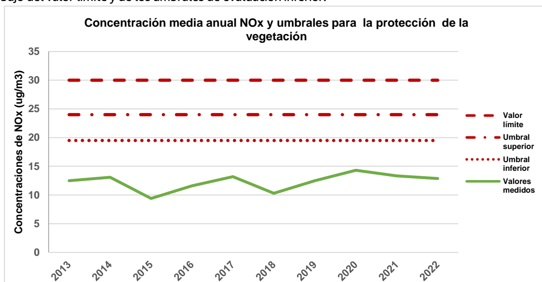
Figura 17. Evolución anual NO x para la protección de la vegetación
