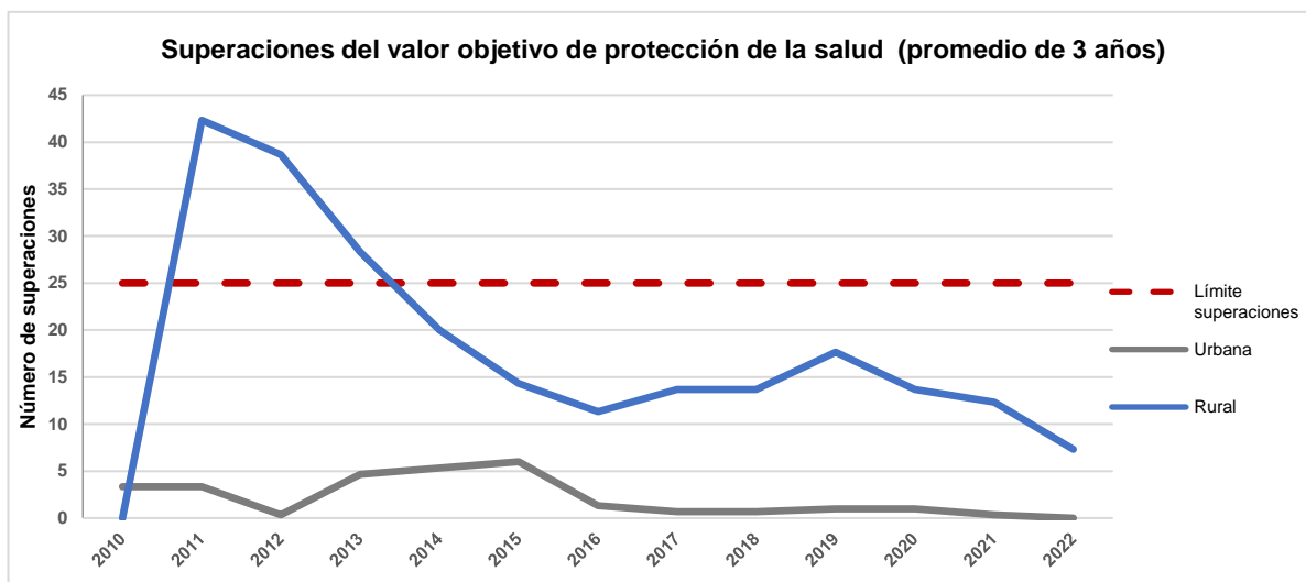
Figura 22. Evolución anual O 3 de las superaciones para la protección de la salud
