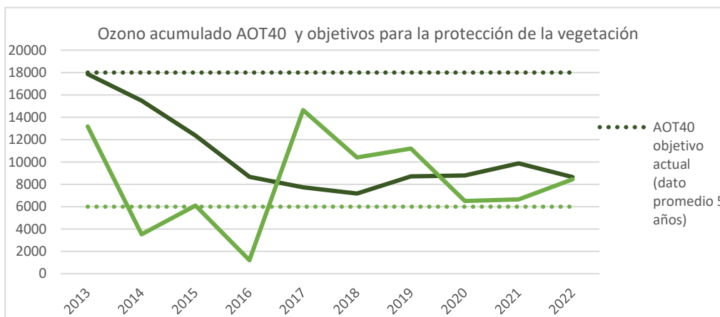
Figura 24. Evolución O 3 para la protección de la vegetación
