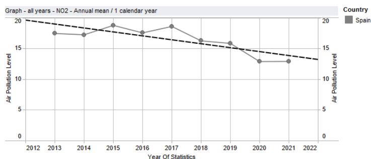
Figura 9. Comparativa de gráficos, de las medias anuales de concentración de NO2 durante los últimos años, de Logroño respecto a España respectivamente. Fuente: European Environment Agency.
