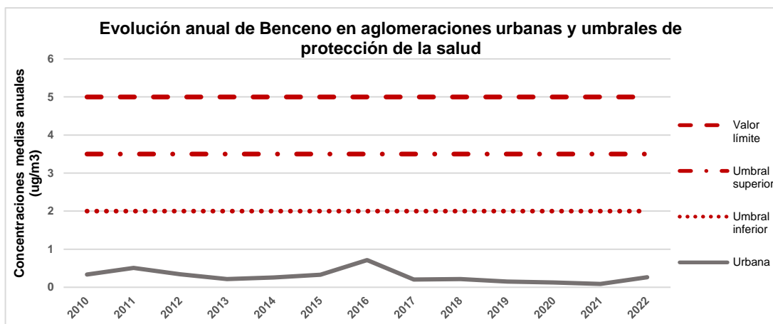
Figura 26. Evolución anual C6H6 para la protección de la salud en zona urbana
