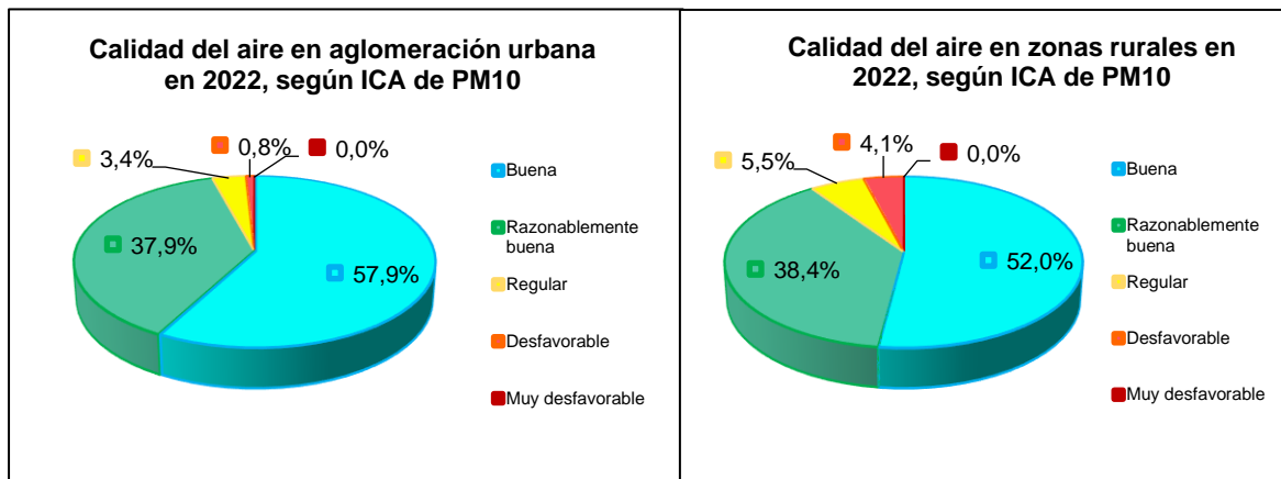
Figura 19. Índice Nacional de Calidad de Aire para PM10 en 2022
