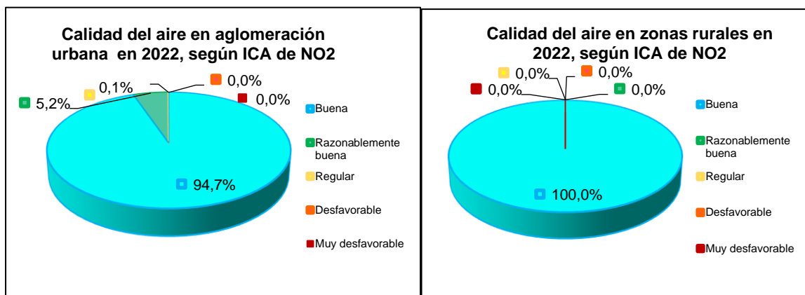
Figura 16. Índice Nacional de Calidad de Aire para NO 2 en 2022
