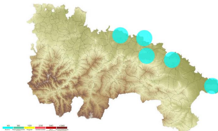
Figura 2. Estaciones de calidad del aire
