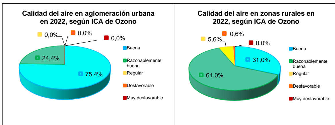
Figura 23. Índice Nacional de Calidad de Aire para O 3 en 2022
