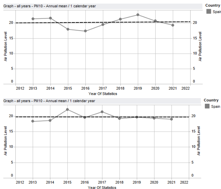
Figura 10. Comparativa de gráficos, de las medias anuales de concentración de PM10 durante los últimos años, de Logroño respecto a España respectivamente. Fuente: European Environment Agency.
