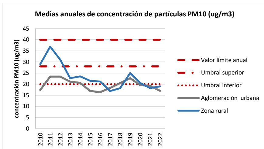
Figura 18. Evolución del promedio anual PM 10 para la protección de la salud. Descontados los episodios naturales por intrusiones Saharianas.
