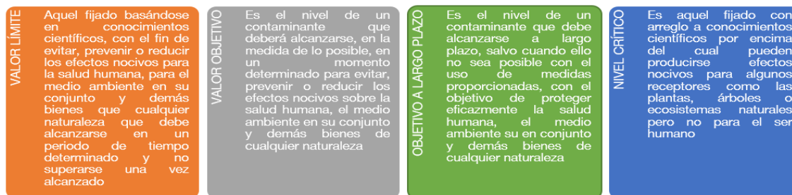
Figura 12. Esquema de los objetivos de calidad y sus definiciones
