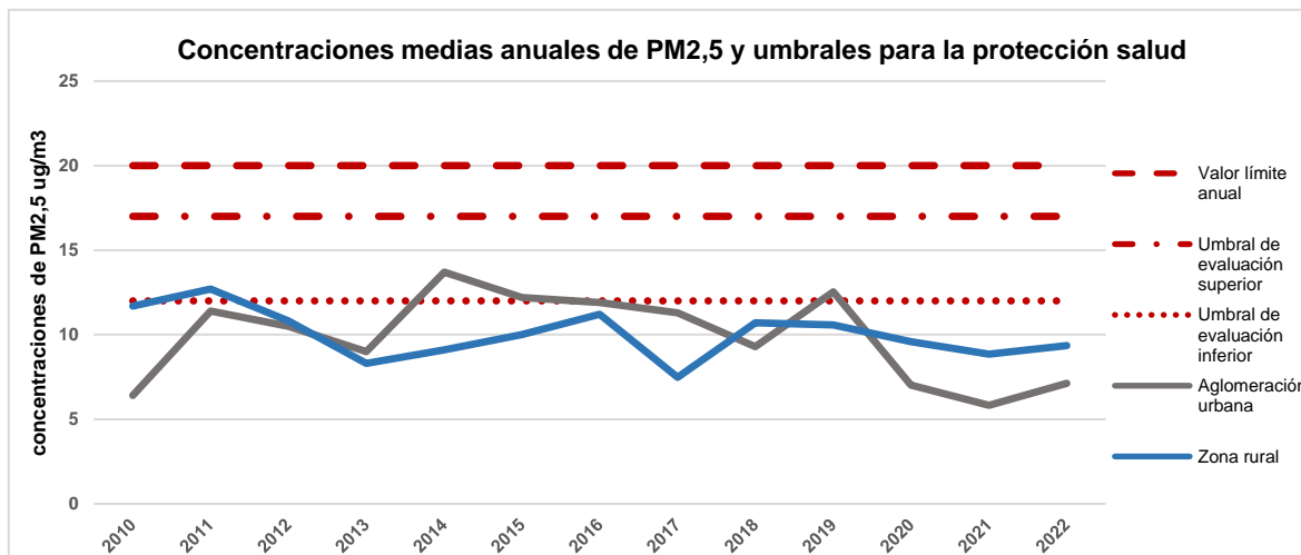
Figura 20. Evolución anual PM 2,5 para la protección de la salud
