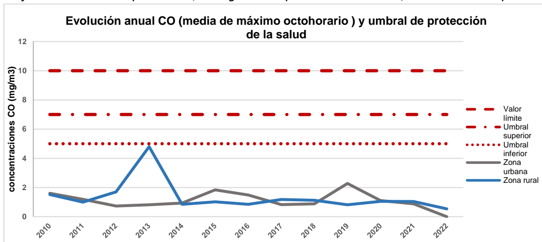
Figura 25. Evolución anual CO para la protección de la salud
