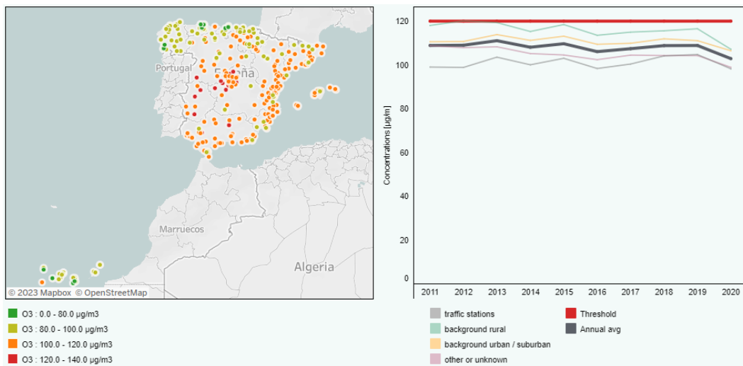
Figura 8. Mapa de las estaciones de medición y gráfico de la evolución de las concentraciones medias España. Fuente: European Environment Agency
