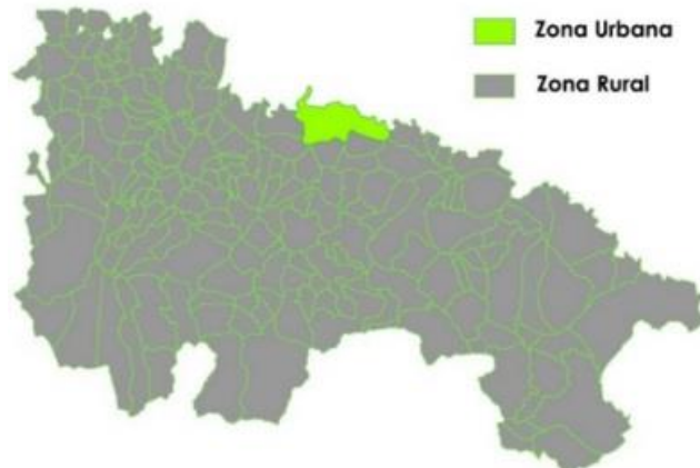
Figura 3. Mapa de La Rioja con la zonificación para la evaluación de la calidad del aire
