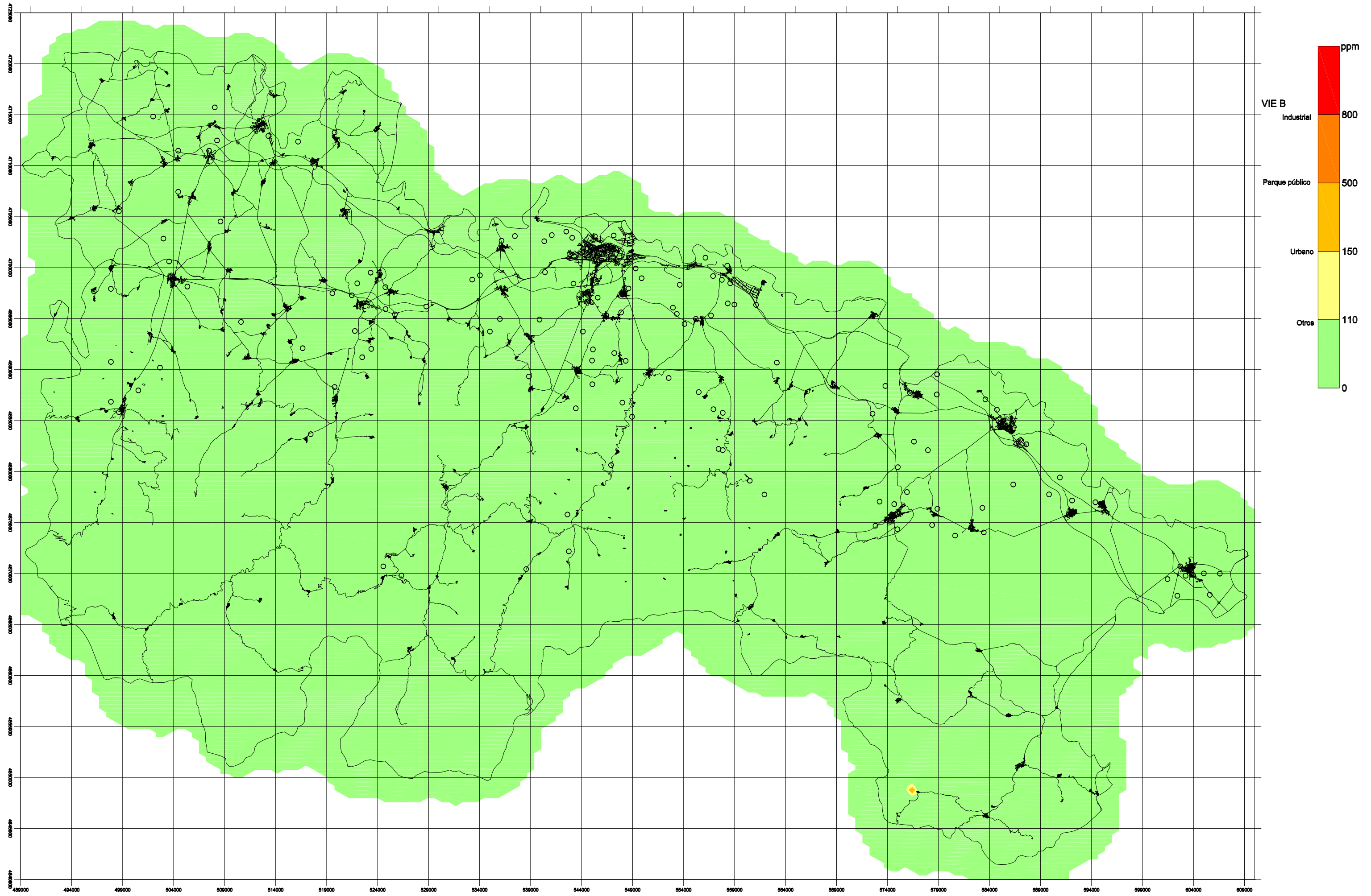
Geoquímica ambiental. Contenidos en el elemento Ni según los límites de contaminación del suelo de la Ley 1/2005 del Gobierno Vasco
