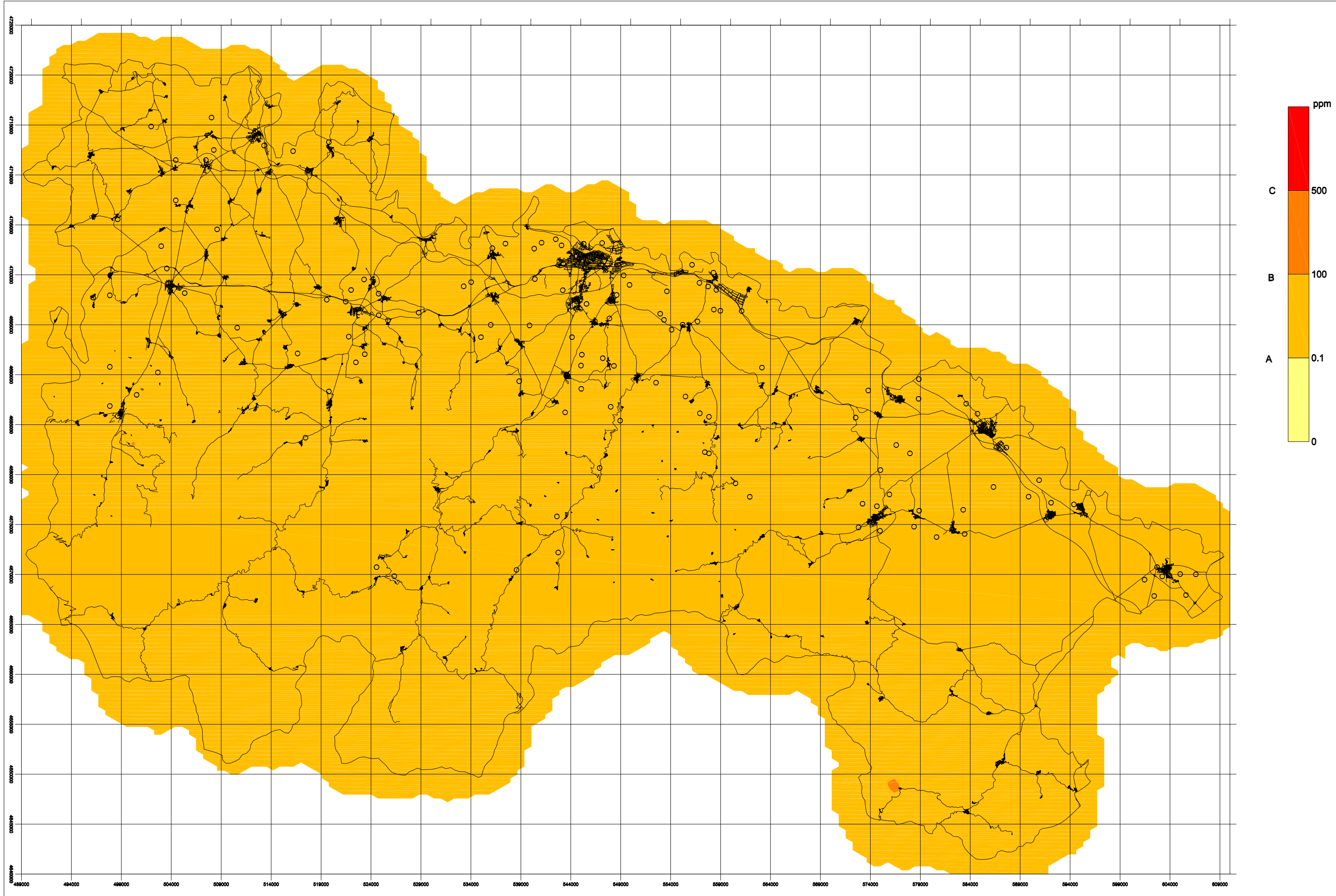
Geoquímica ambiental. Contenidos en el elemento Ni según los límites de contaminación del suelo de la normativa holandesa.
