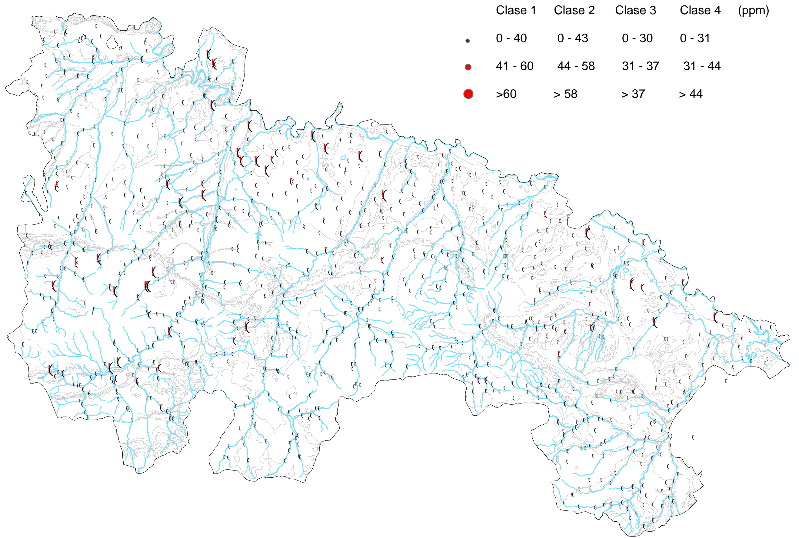
Figura 8.10. Anomalías del Cu por clases geoquímicas
