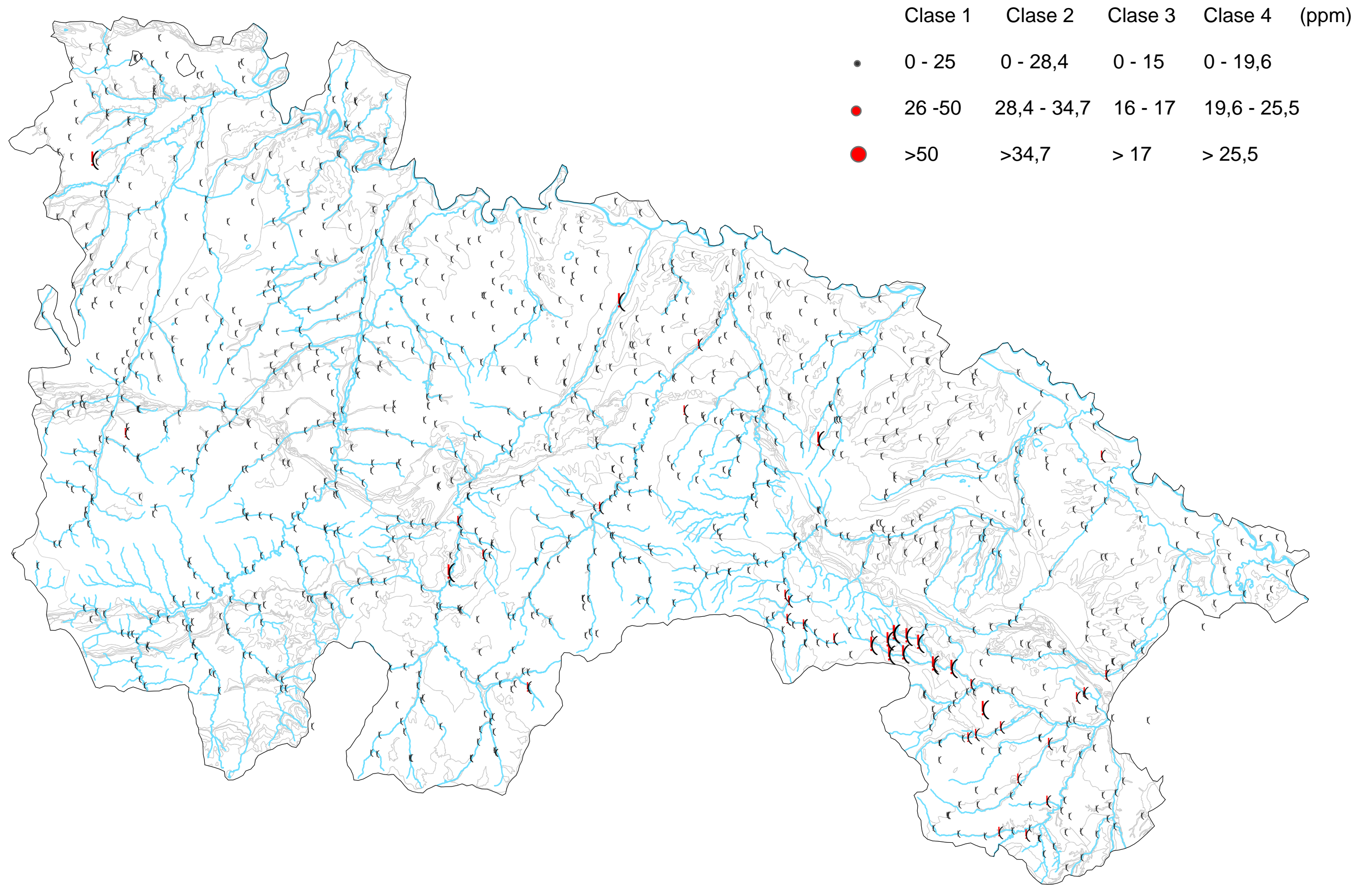
Figura 8.8. Anomalías del As por clases geoquímicas
