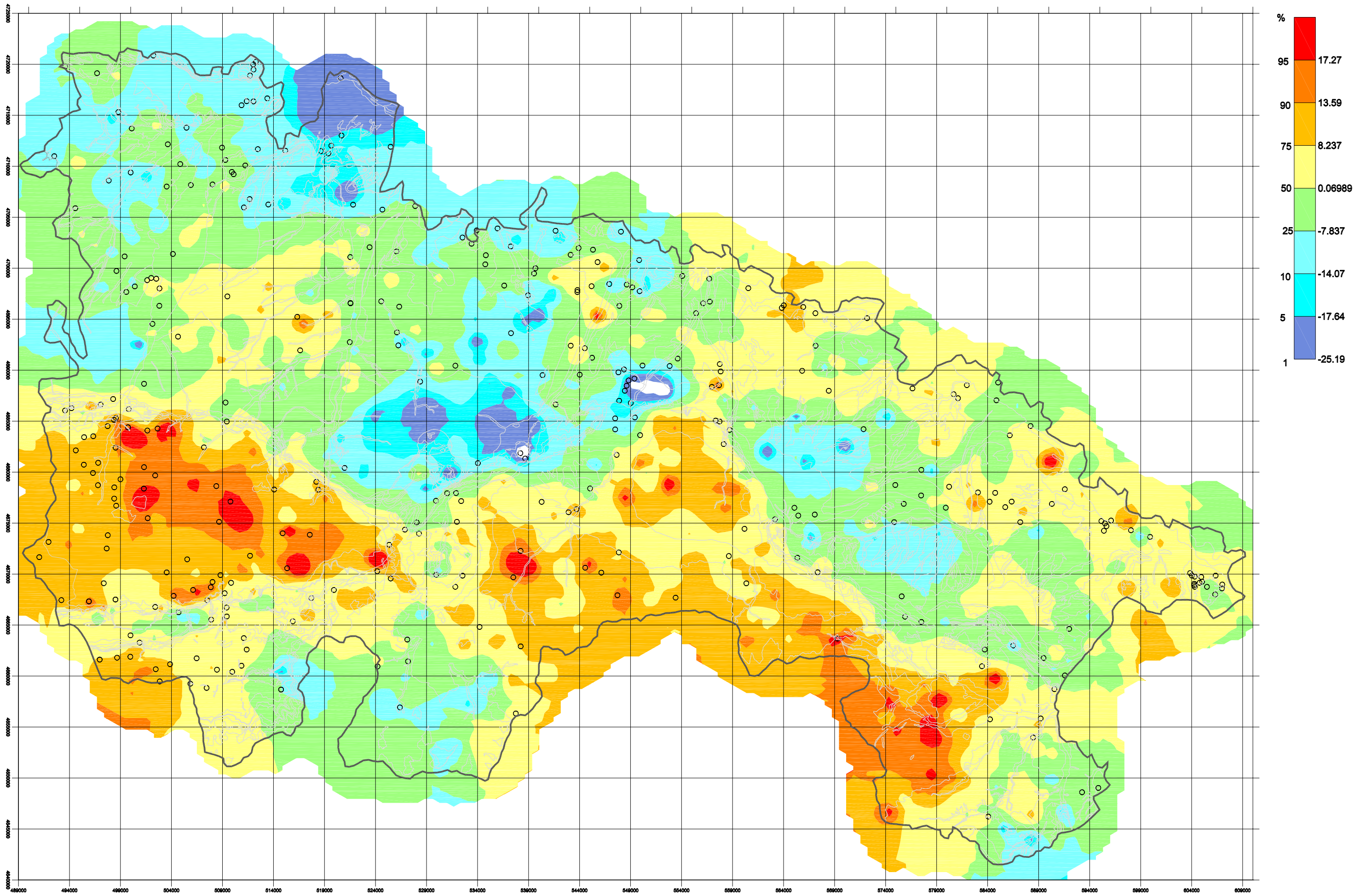
Distribución del componente 1. Sc - Ni - Fe - Cs - V - Cr - Co - Rb - Be - As - Sb - K - (Mn - Zn - Al - U - Pb - La - Cu - Nd - Sm - Th)
