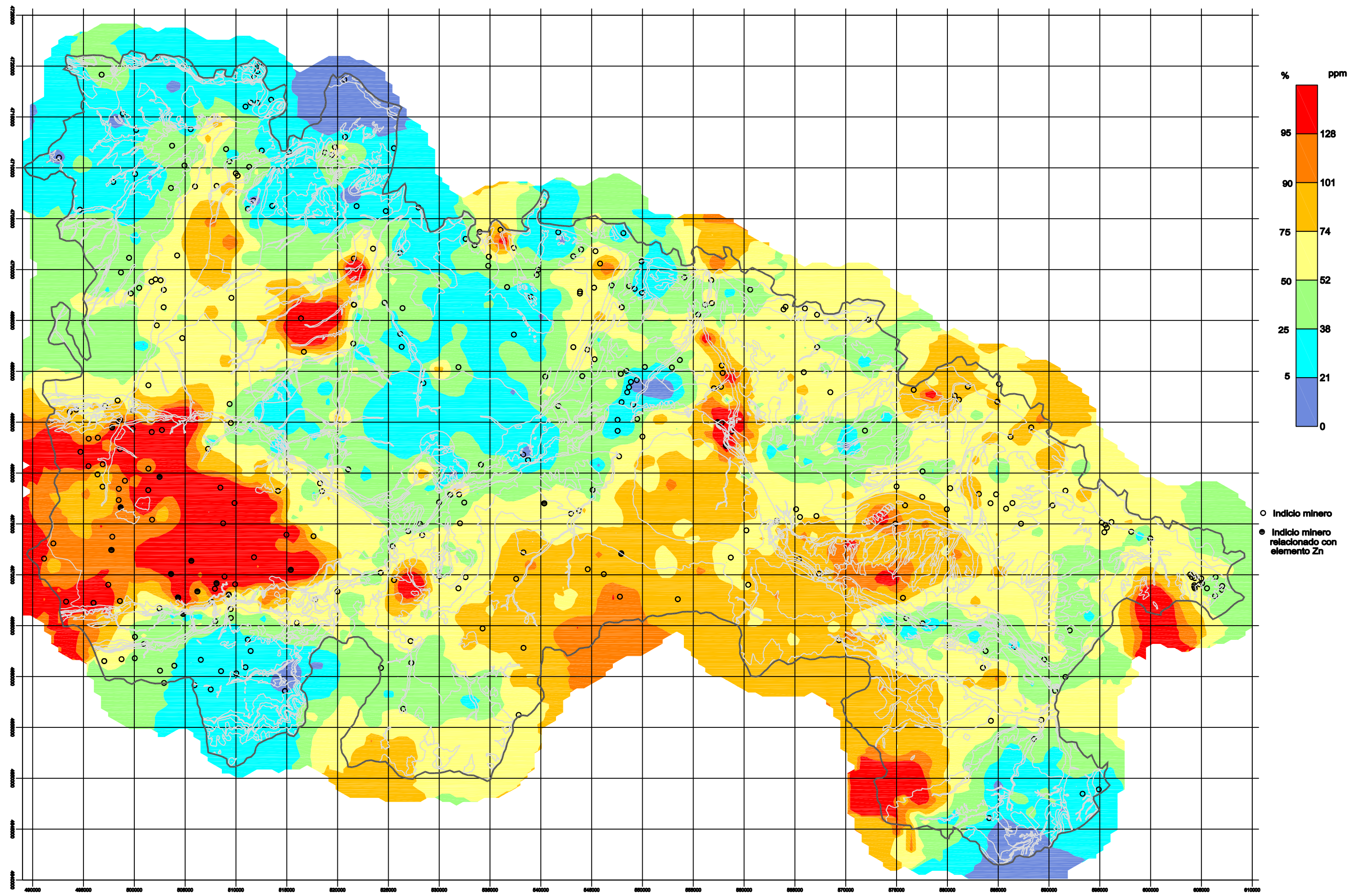
Figura 6.45: Tratamiento geoquímico univariante. Distribución del Zn
