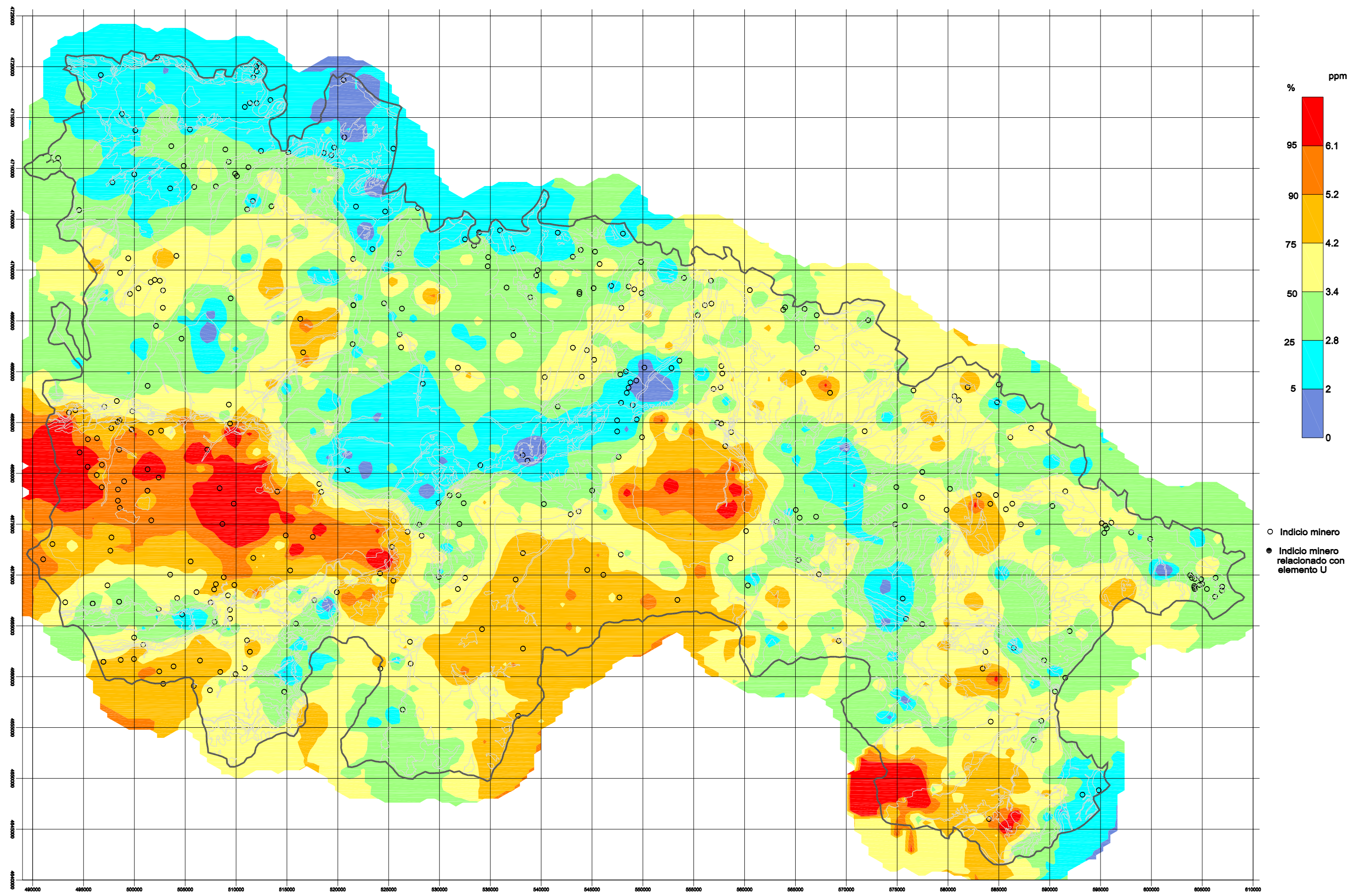
Figura 6.40: Tratamiento geoquímico univariante. Distribución del U
