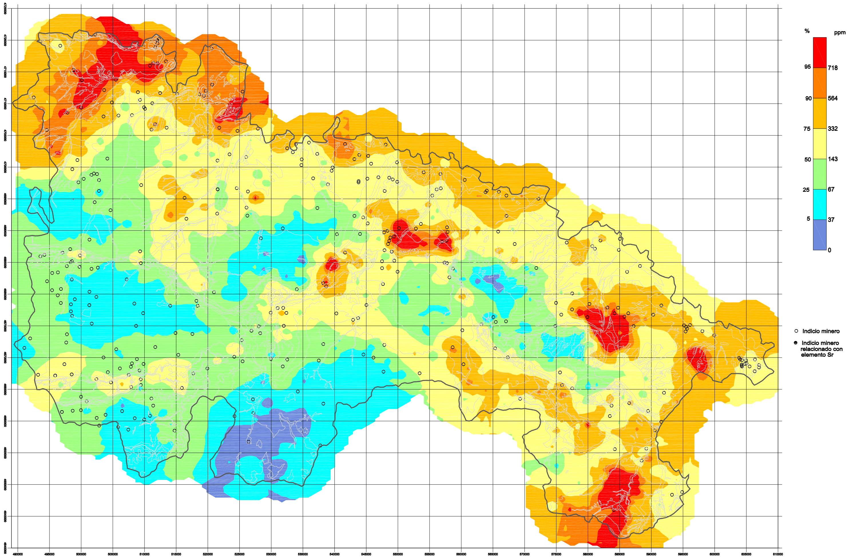
Figura 6.35: Tratamiento geoquímico univariante. Distribución del Sr
