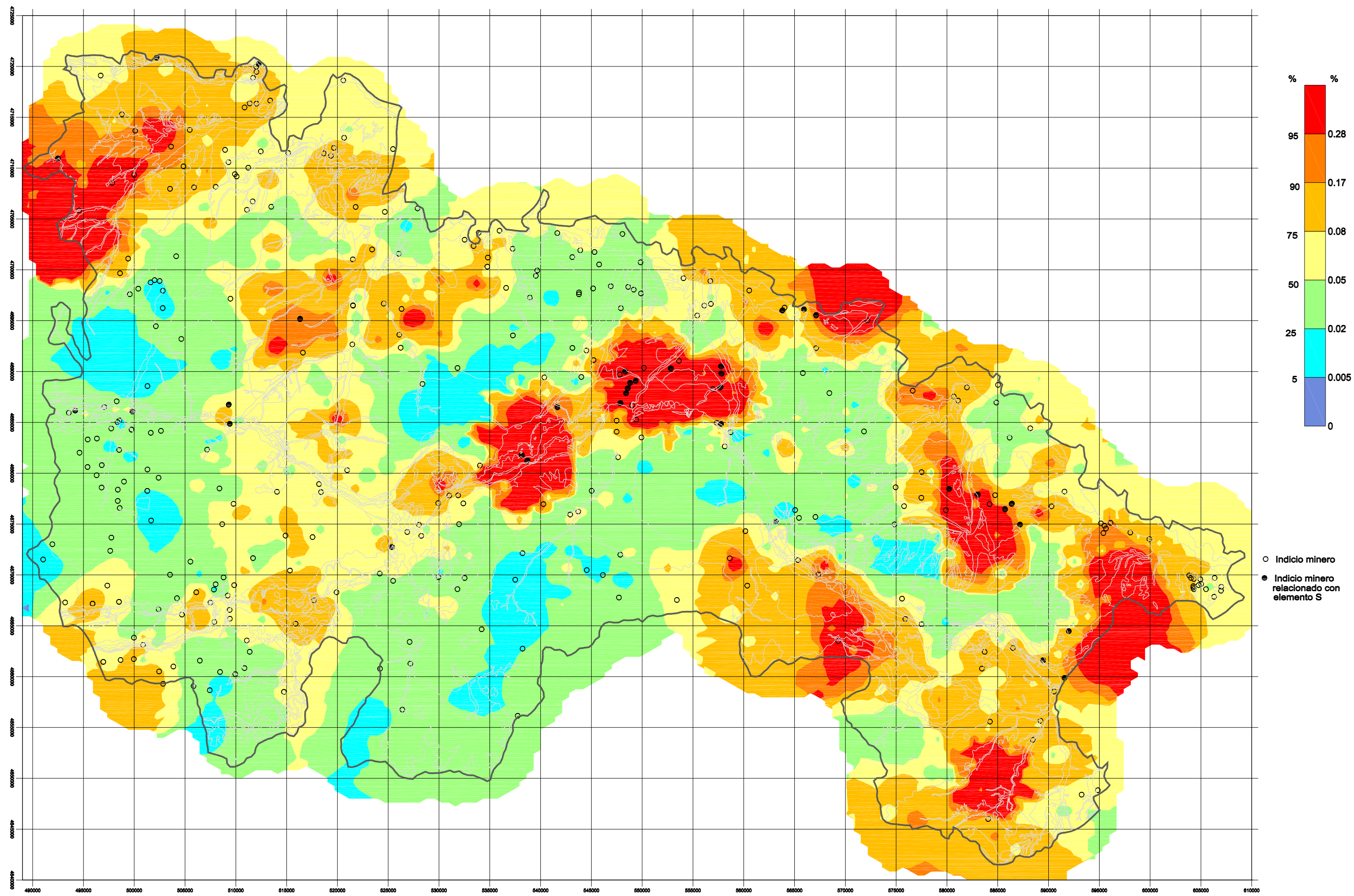
Figura 6.31: Tratamiento geoquímico univariante. Distribución del S
