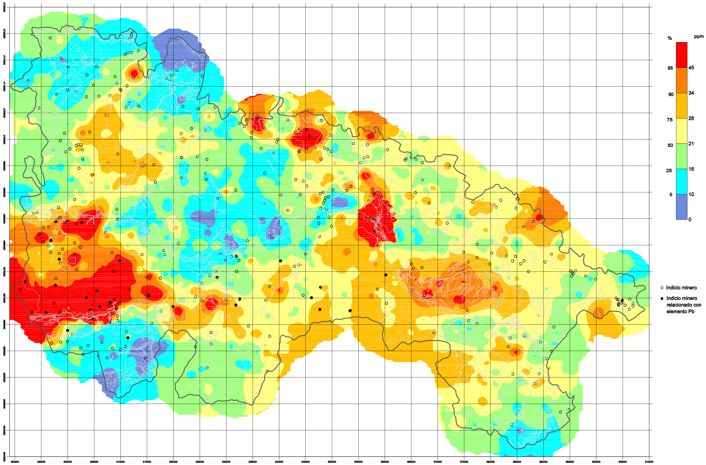
Figura 6.29: Tratamiento geoquímico univariante. Distribución del Pb
