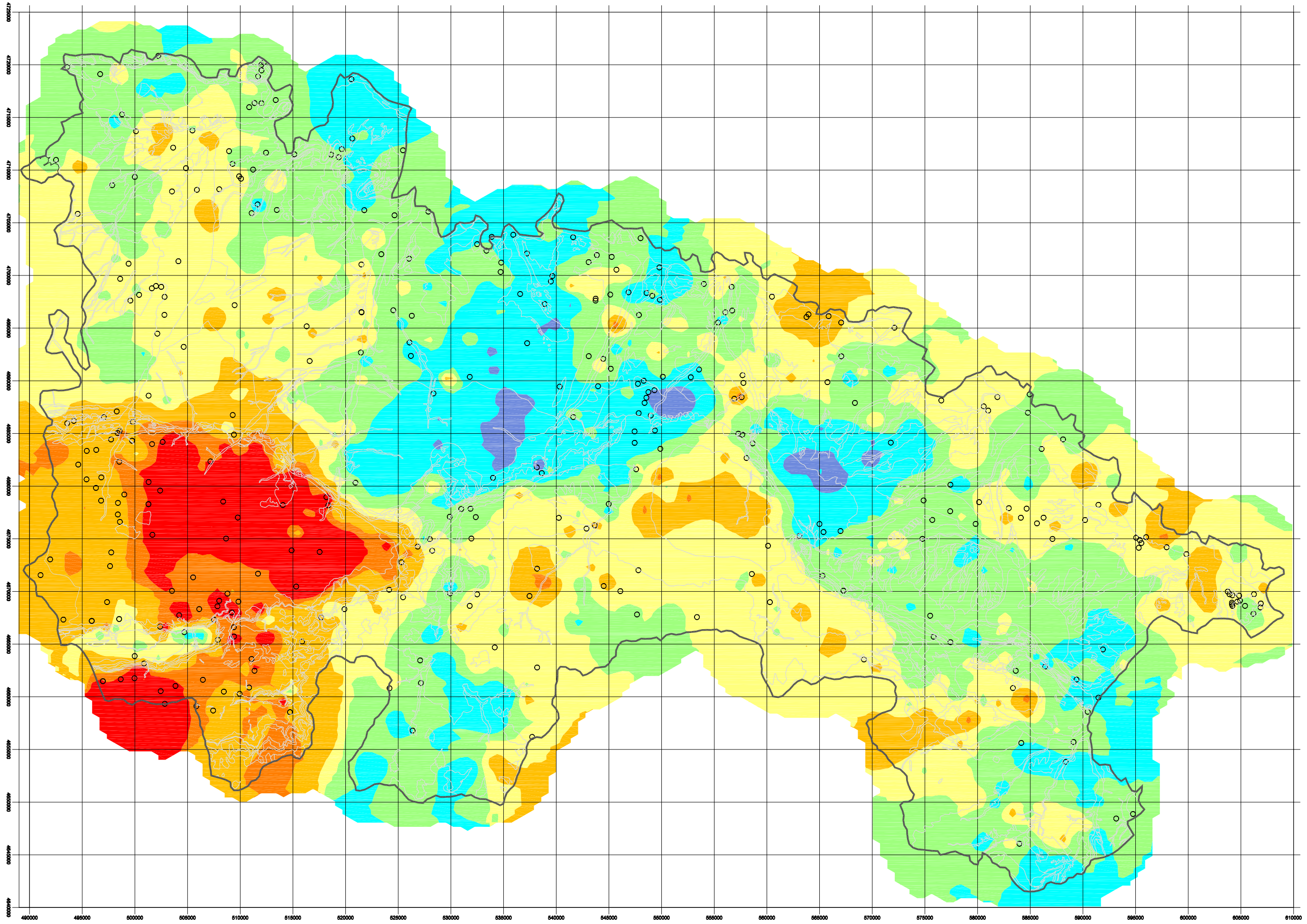
Figura 6.19: Tratamiento geoquímico univariante. Distribución del K
