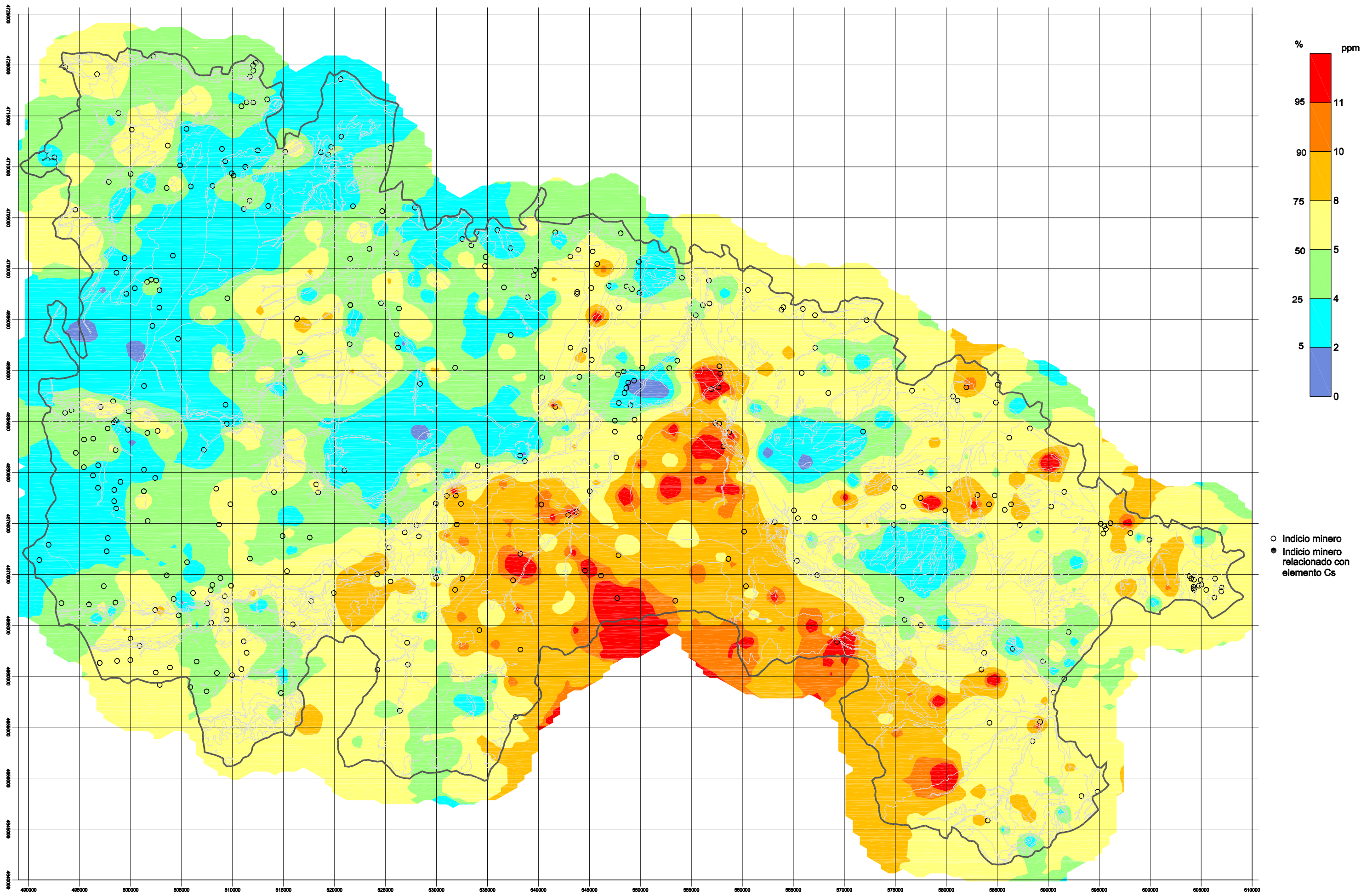
Figura 6.14: Tratamiento geoquímico univariante. Distribución del Cs
