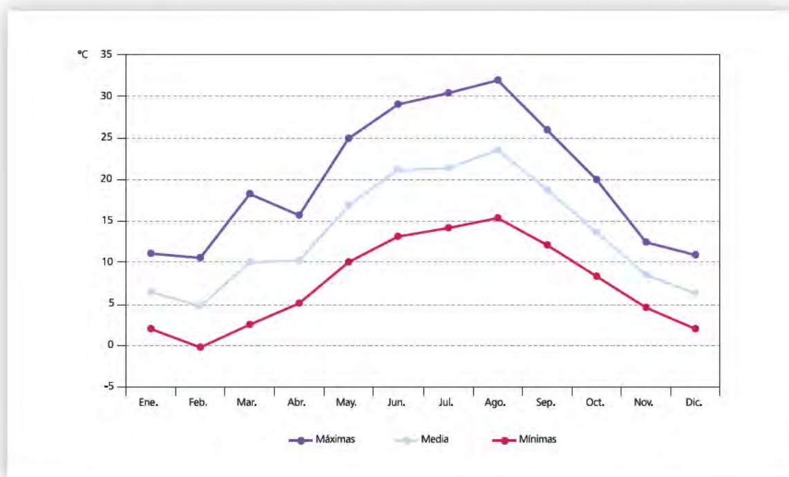
GRÁFICO 1.2. TEMPERATURAS MEDIAS MENSUALES EN LOGROÑO. OBSERVATORIO DE AGONCILLO. 2012
