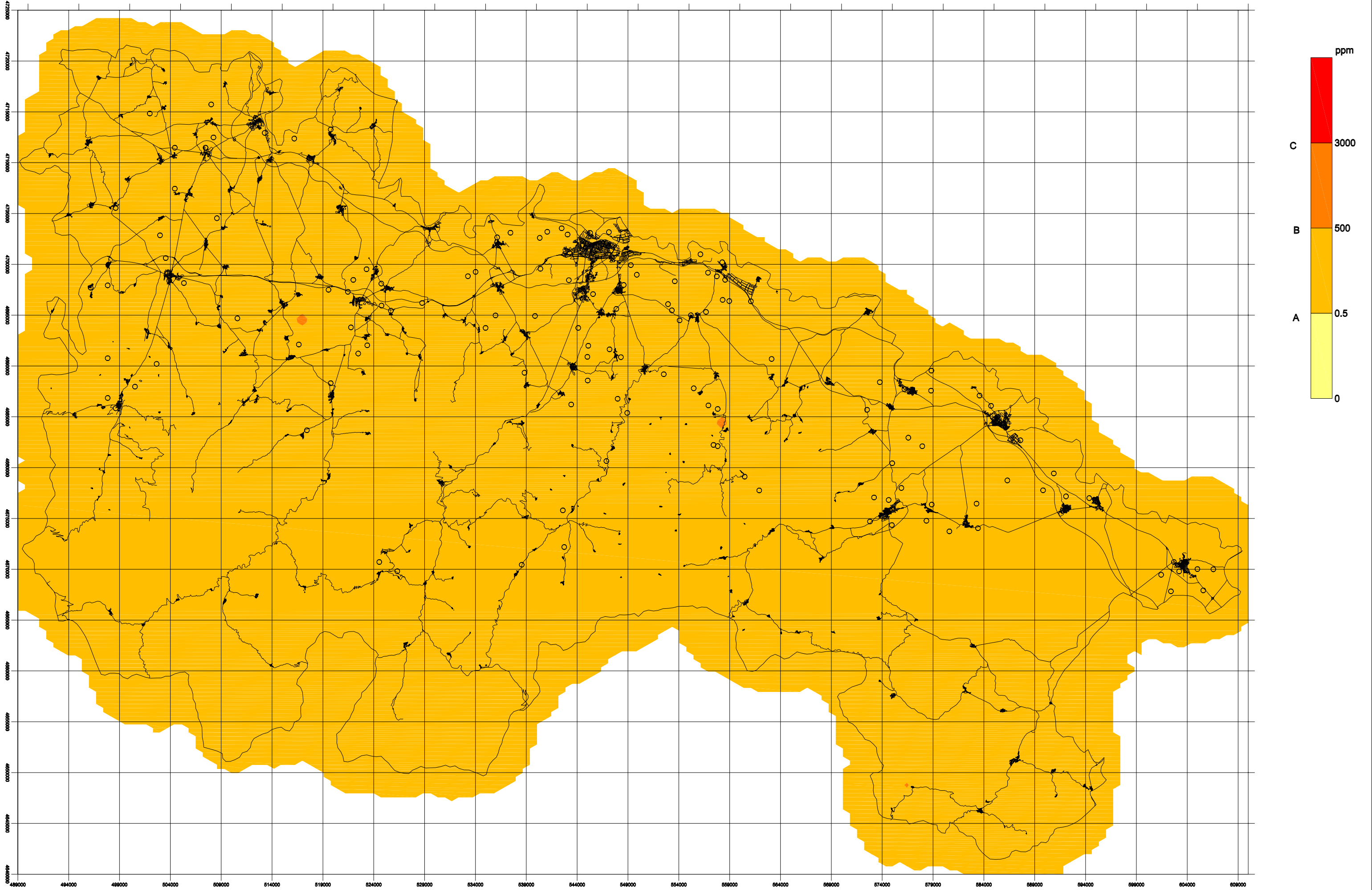
Geoquímica ambiental. Contenidos en el elemento Zn según los límites de contaminación del suelo de la normativa holandesa.
