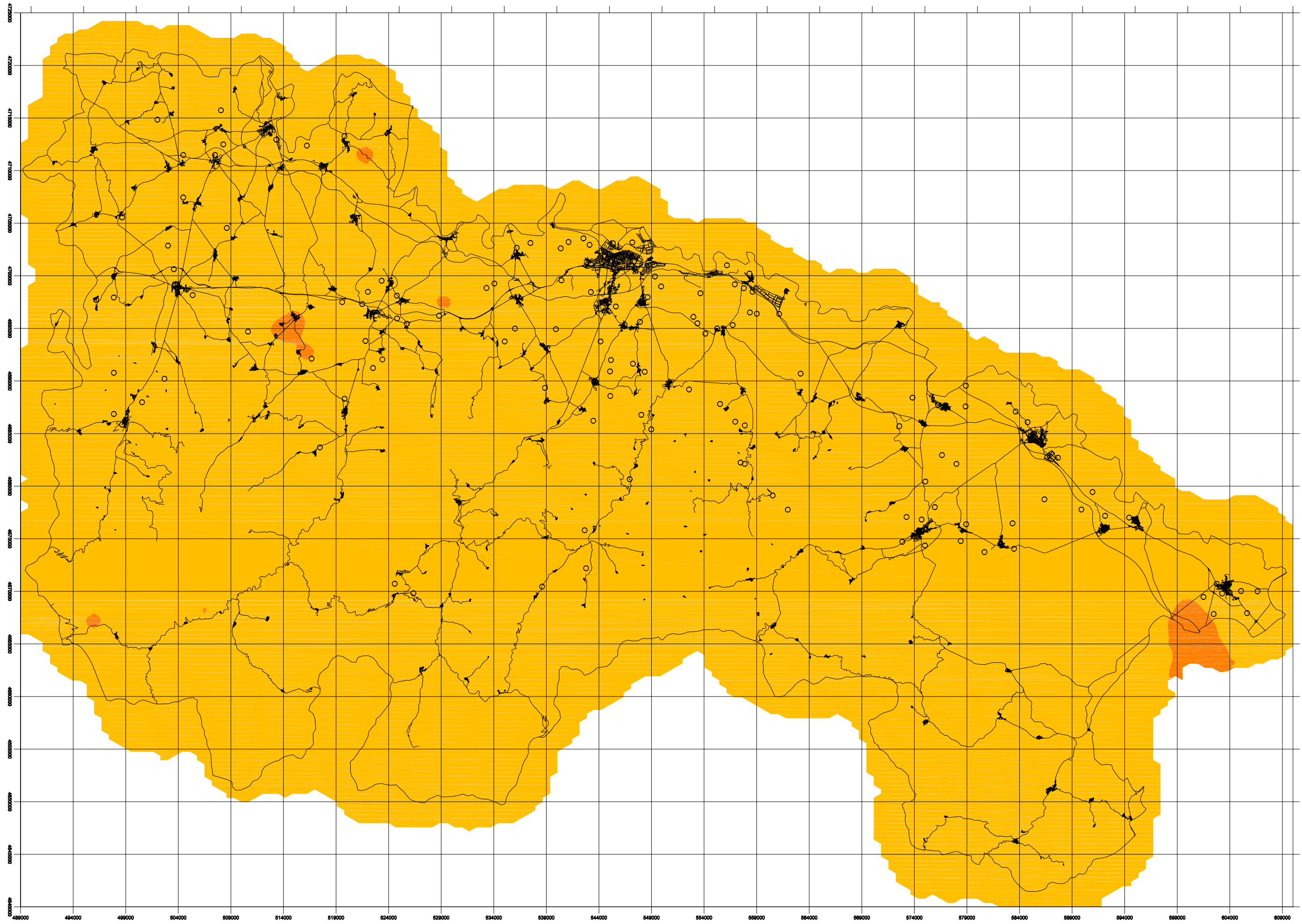
Geoquímica ambiental. Contenidos en el elemento Cu según los límites de contaminación del suelo de la normativa holandesa.
