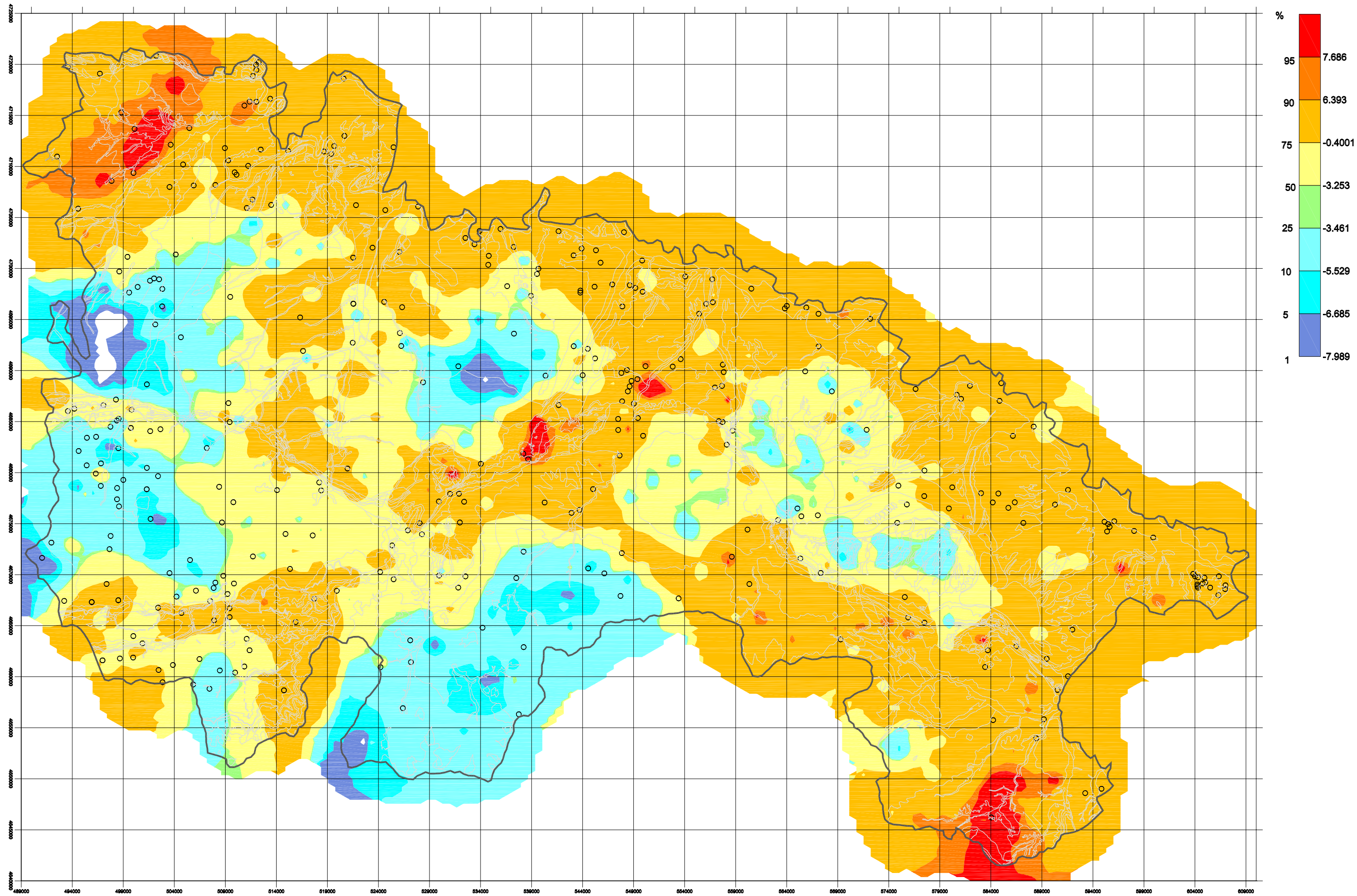
Distribución del componente 3. Sr - S - Ca - Mg - (P - Br)
