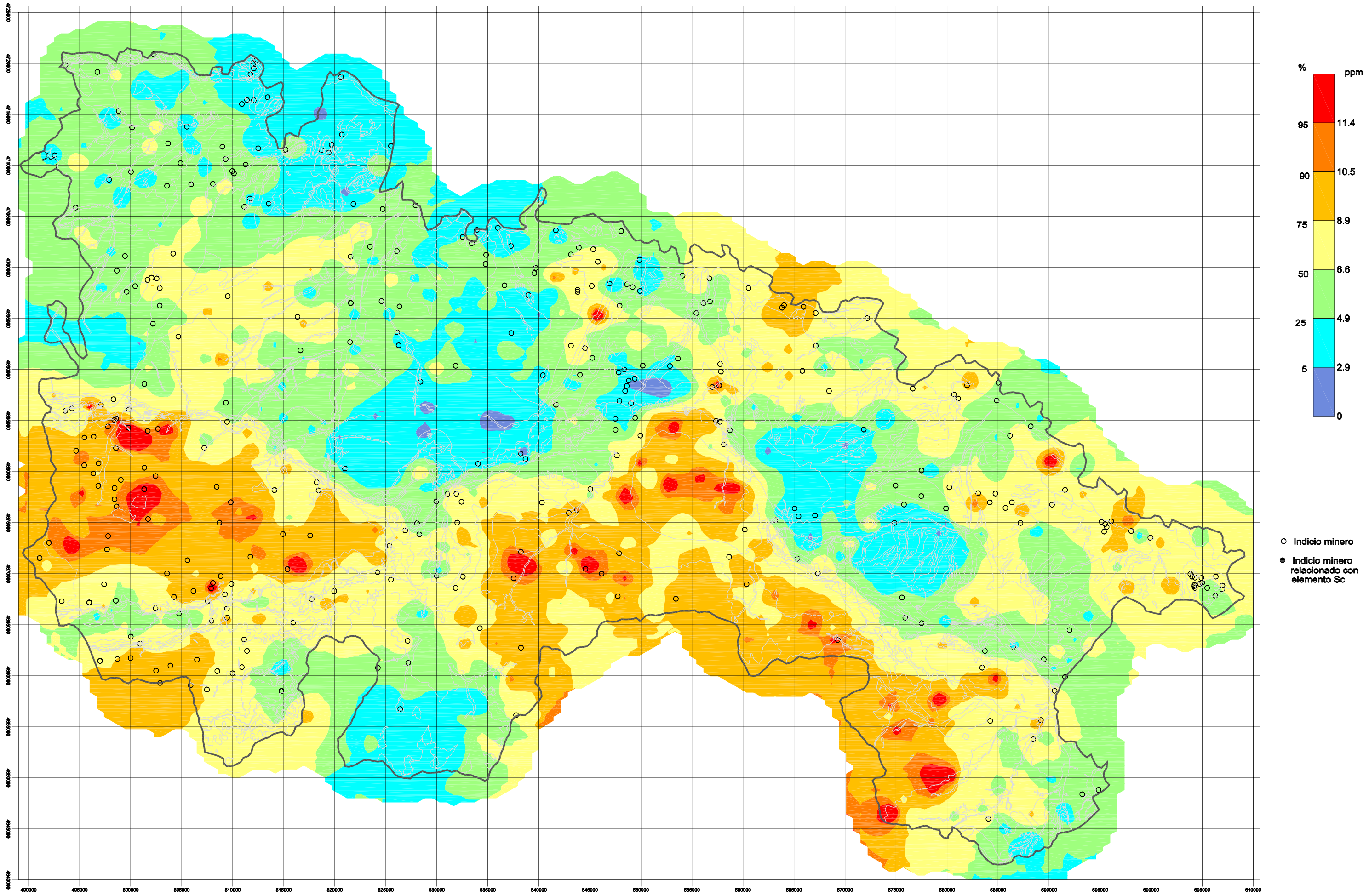
Figura 6.33: Tratamiento geoquímico univariante. Distribución del Sc
