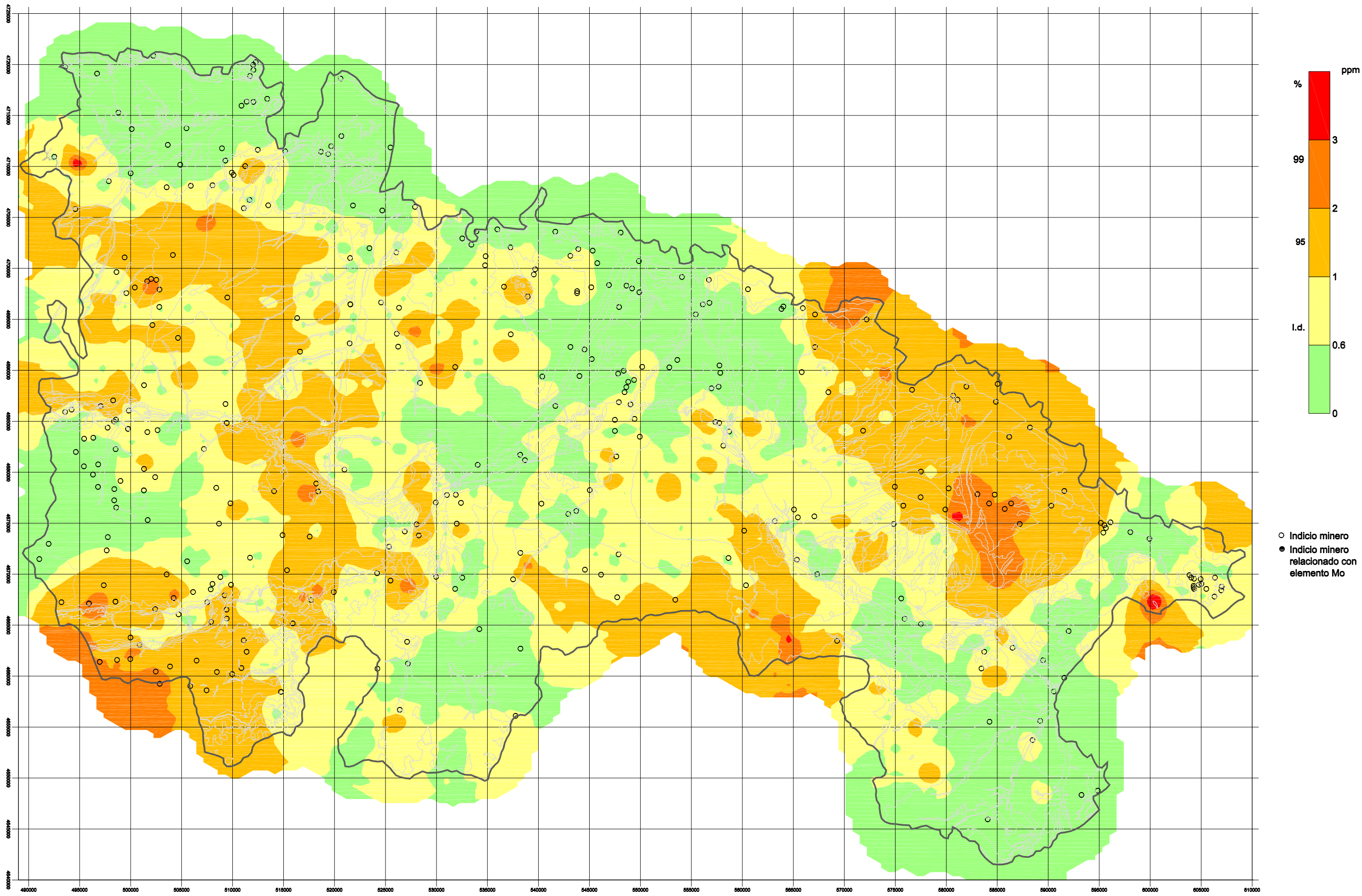
Figura 6.24: Tratamiento geoquímico univariante. Distribución del Mo
