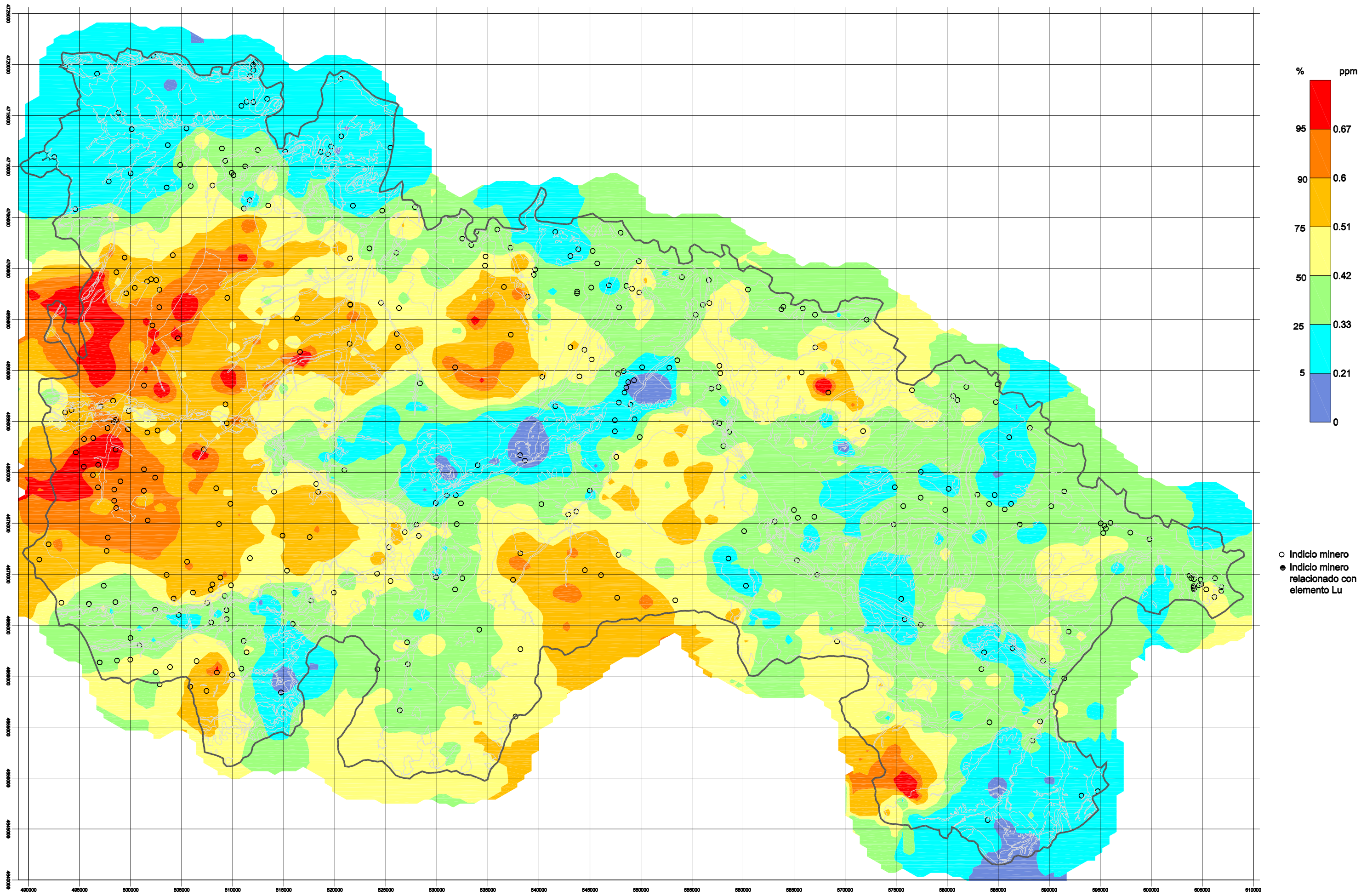
Figura 6.21: Tratamiento geoquímico univariante. Distribución del Lu
