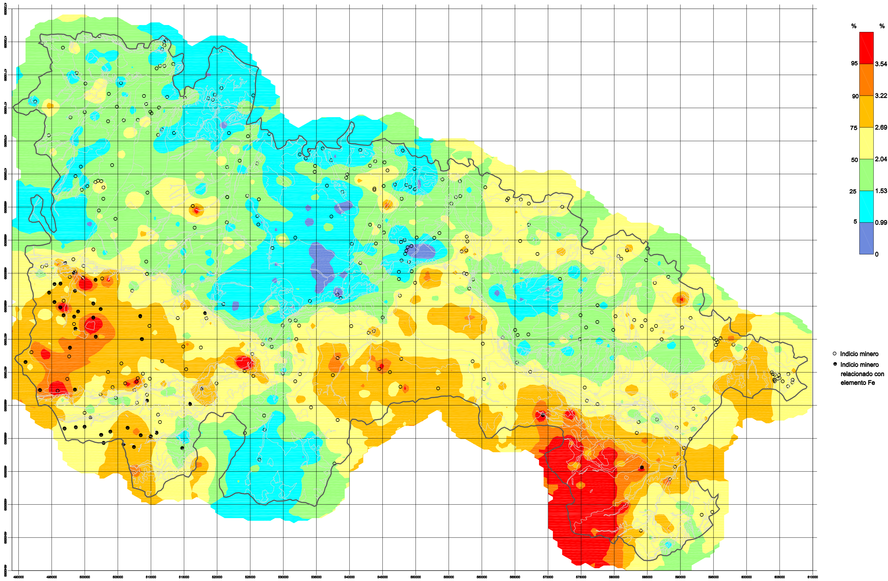
Figura 6.17: Tratamiento geoquímico univariante. Distribución del Fe
