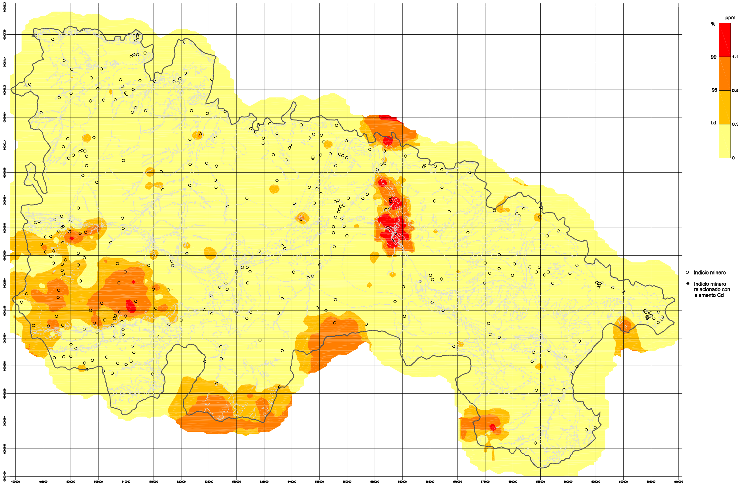
Figura 6.10: Tratamiento geoquímico univariante. Distribución del Cd
