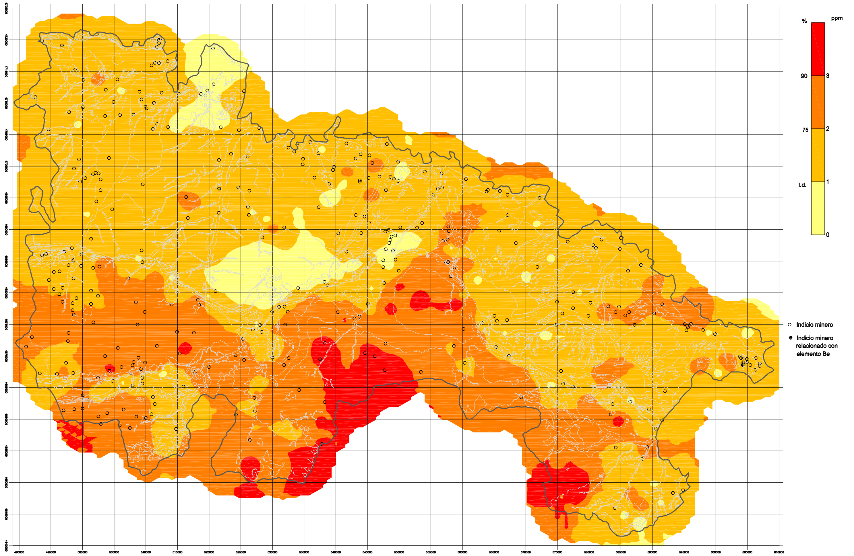
Figura 6.6: Tratamiento geoquímico univariante. Distribución del Be
