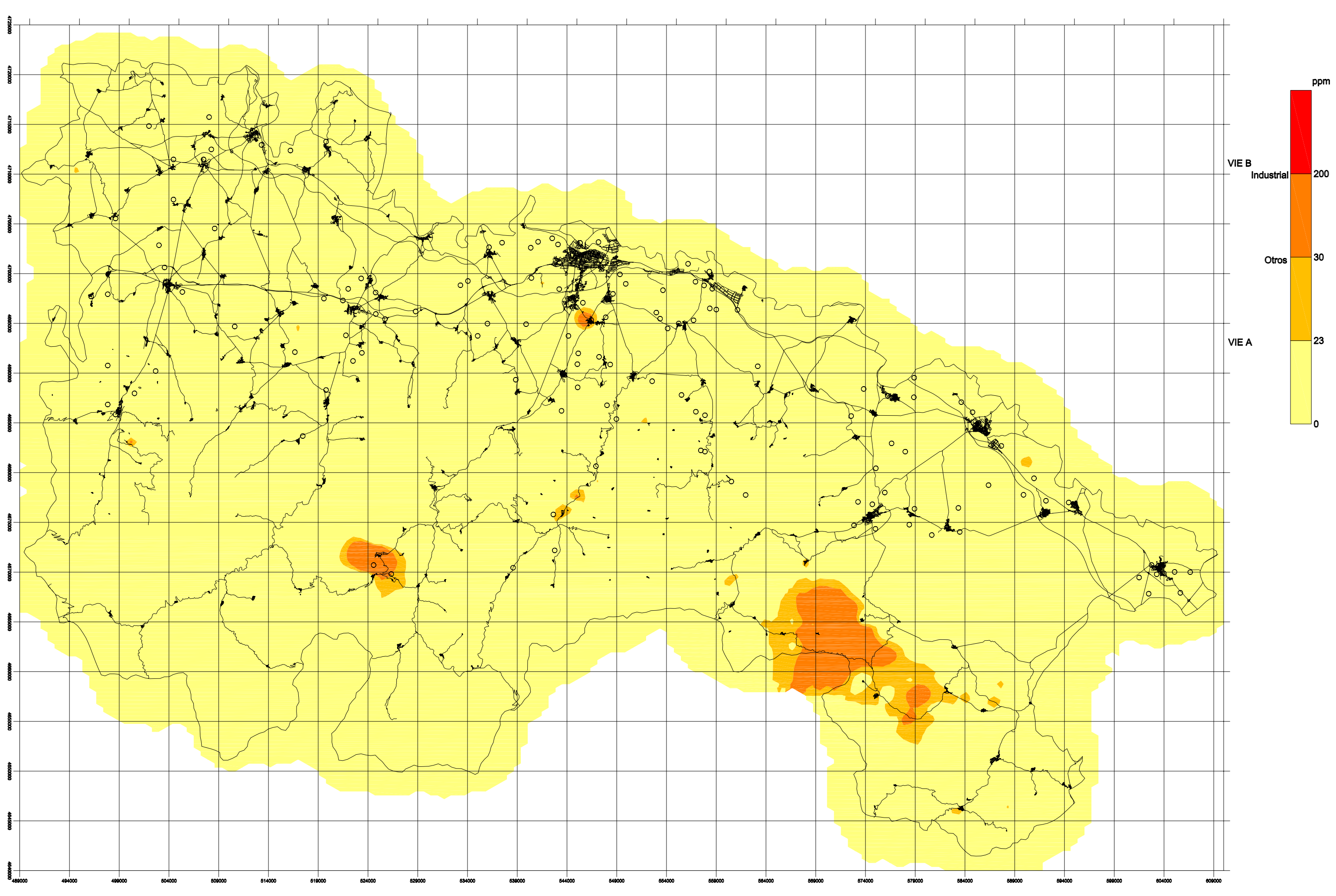
Geoquímica ambiental. Contenidos en el elemento As según los límites de contaminación del suelo de la Ley 1/2005 del Gobierno Vasco
