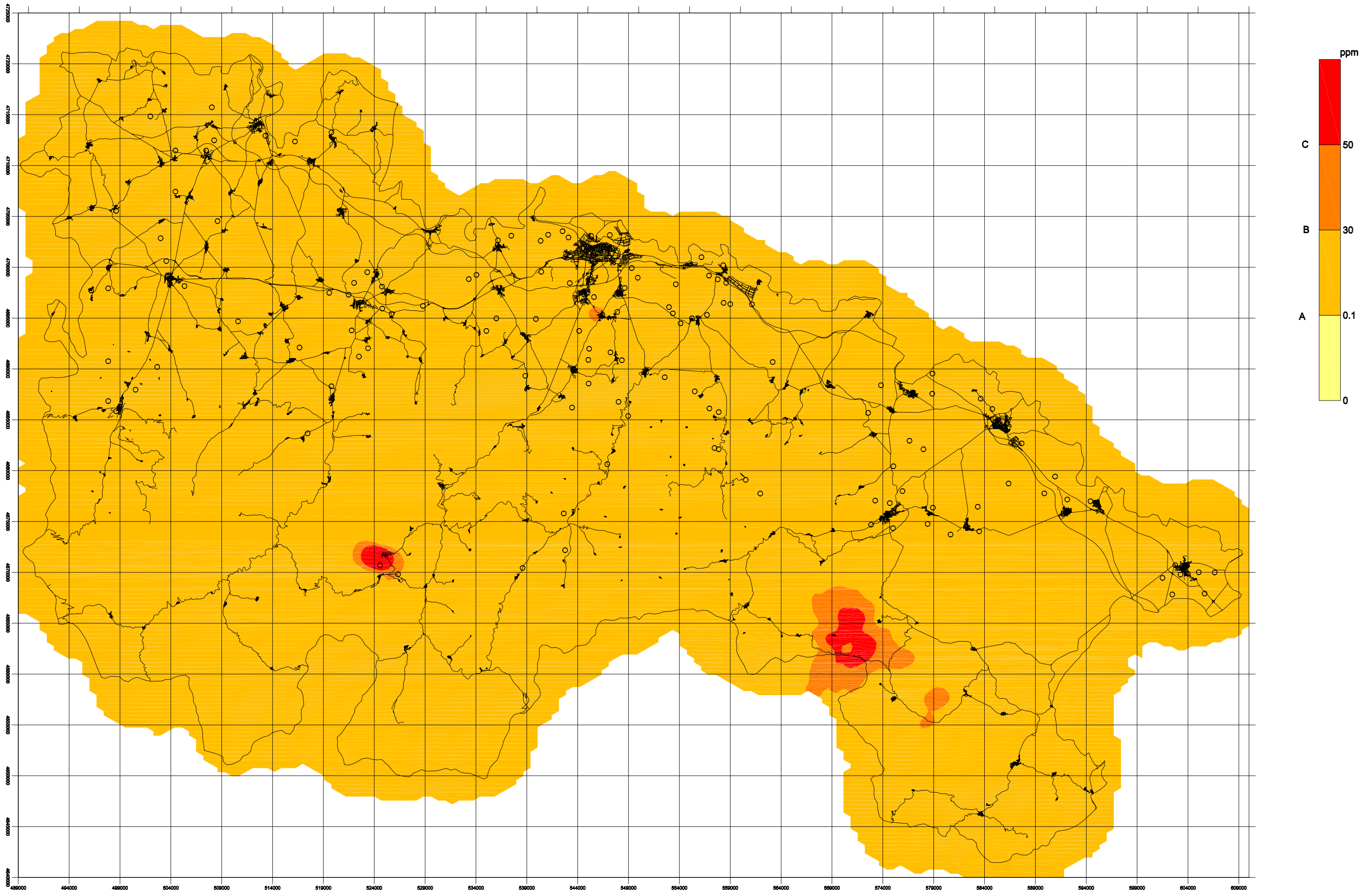
Geoquímica ambiental. Contenidos en el elemento As según los límites de contaminación del suelo de la normativa holandesa.
