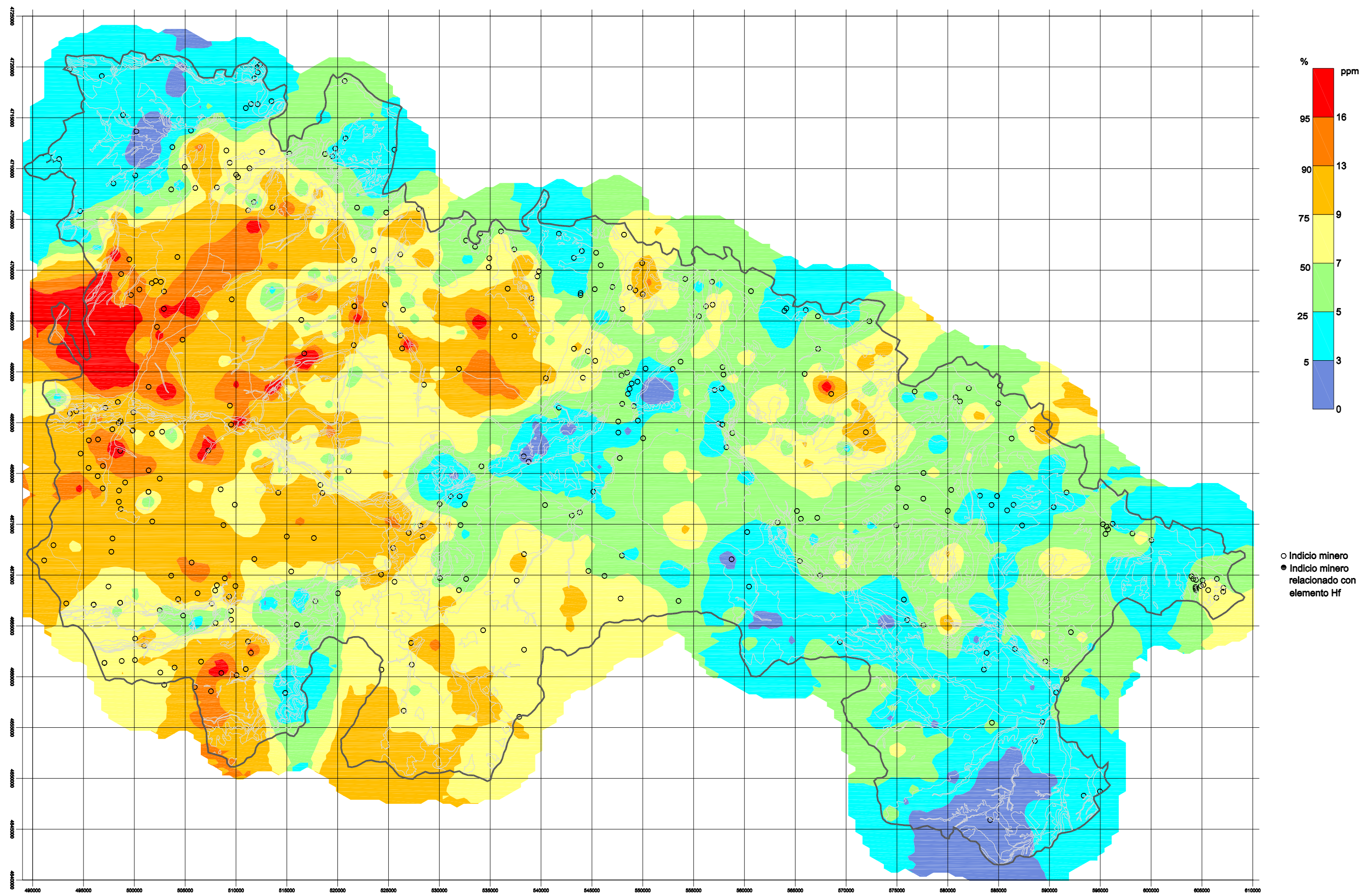
Figura 6.18: Tratamiento geoquímico univariante. Distribución del Hf
