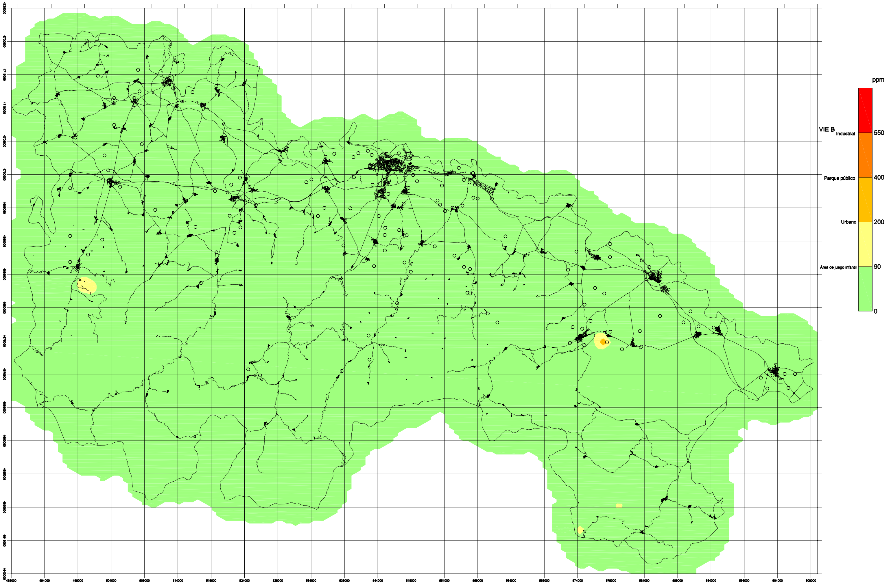
Geoquímica ambiental. Contenidos en el elemento Cr según los límites de contaminación del suelo de la Ley 1/2005 del Gobierno Vasco
