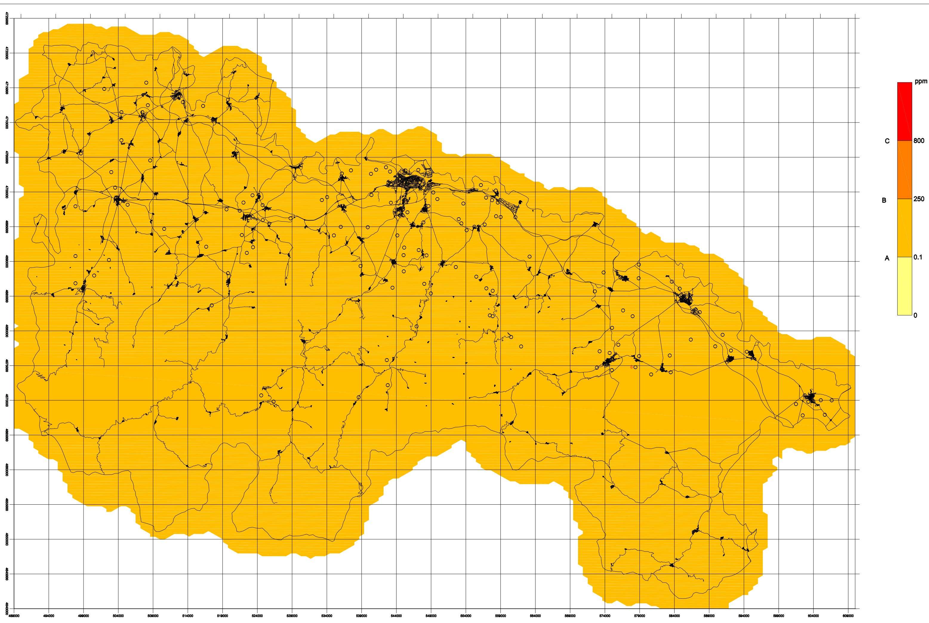
Geoquímica ambiental. Contenidos en el elemento Cr según los límites de contaminación del suelo de la normativa holandesa.
