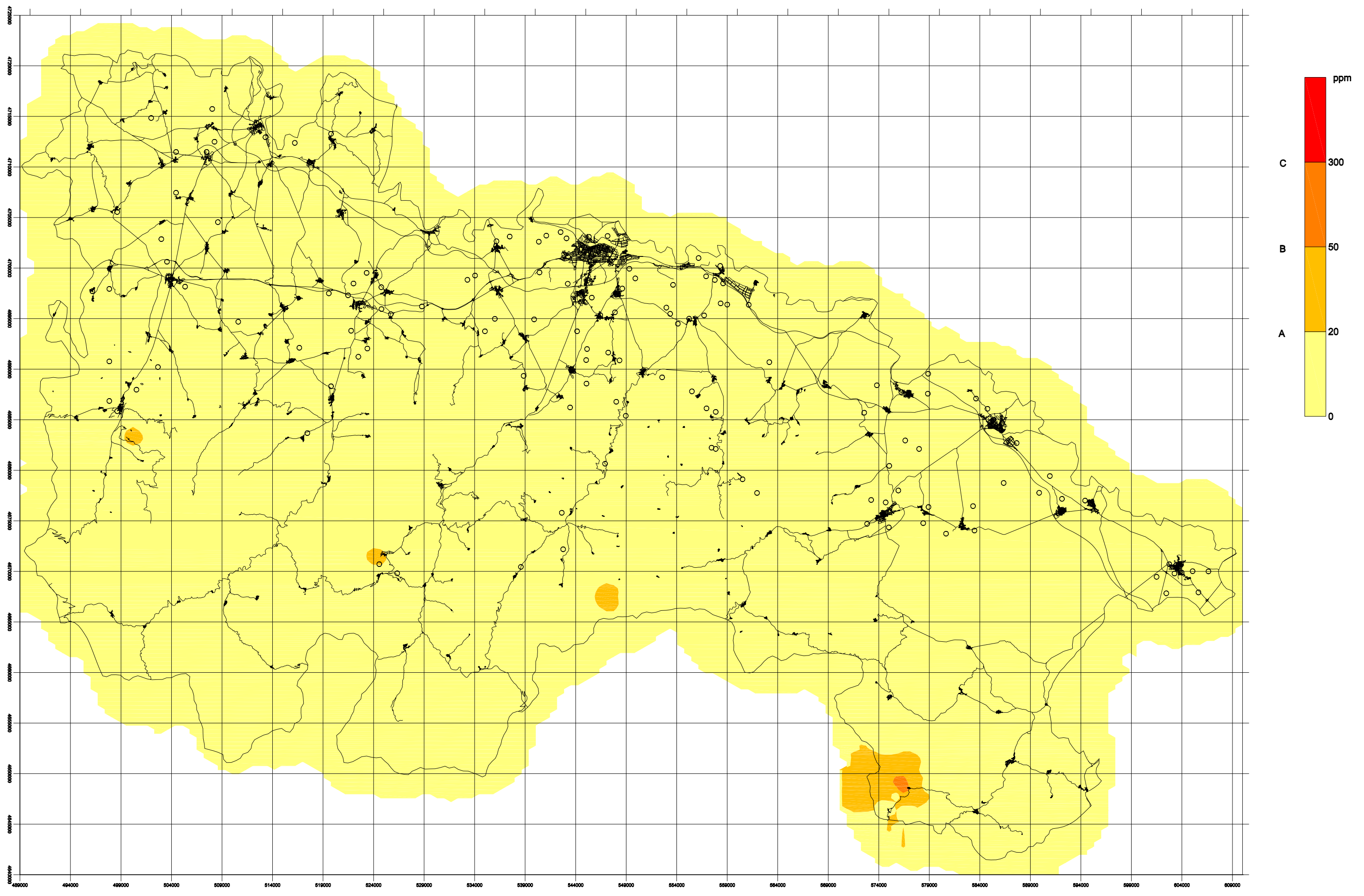
Geoquímica ambiental. Contenidos en el elemento Co según los límites de contaminación del suelo de la normativa holandesa.
