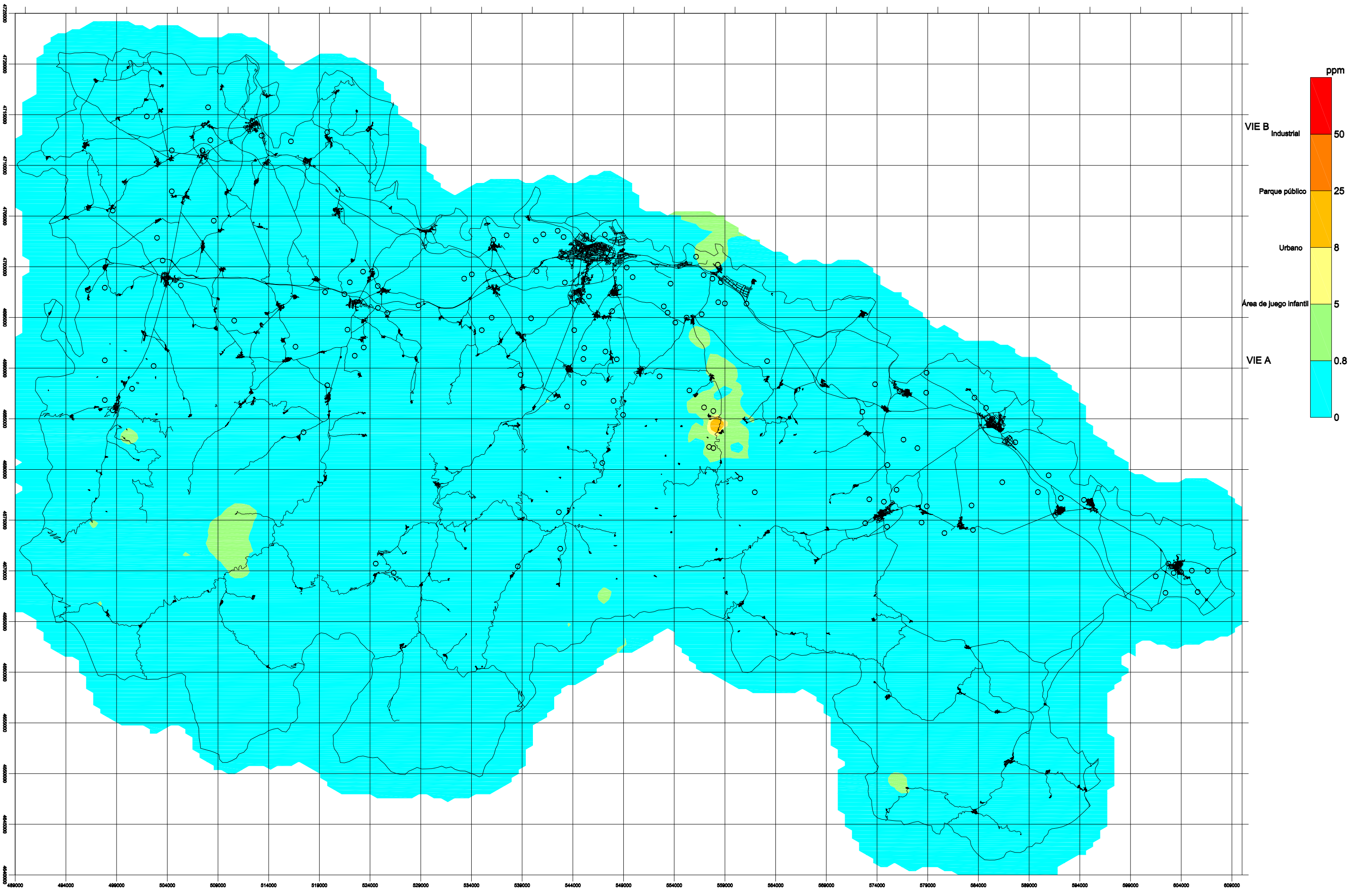
Geoquímica ambiental. Contenidos en el elemento Cd según los límites de contaminación del suelo de la Ley 1/2005 del Gobierno Vasco
