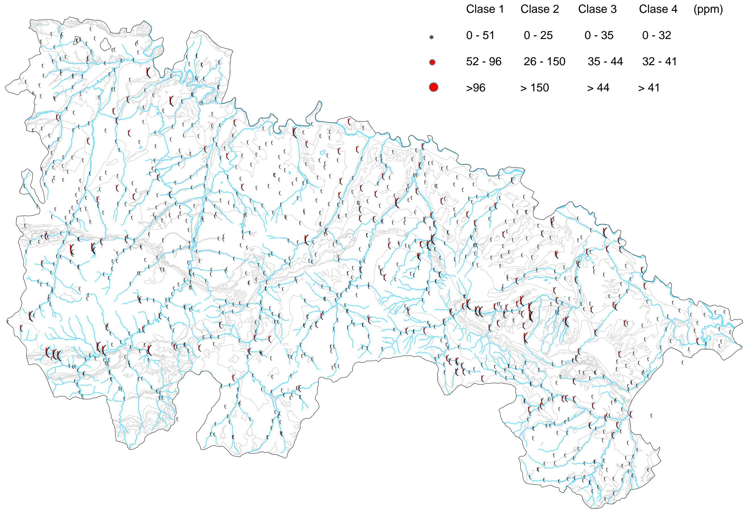
Figura 8.11. Anomalías del Pb por clases geoquímicas
