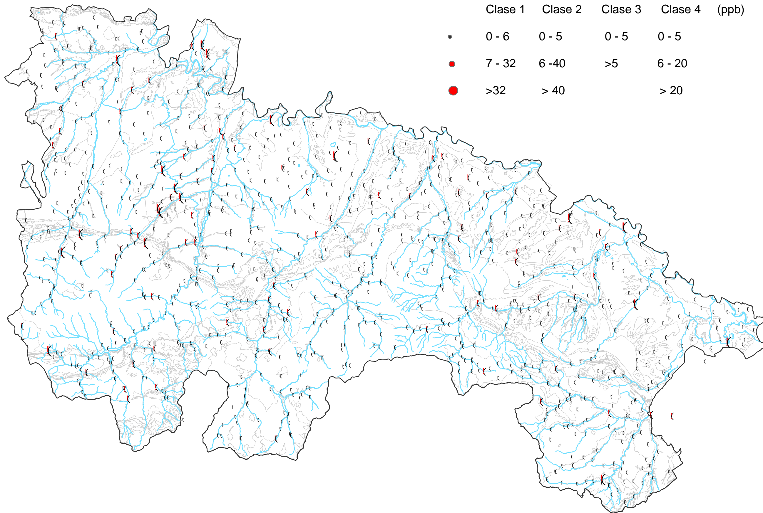
Figura 8.9 Anomalías de Au por clases geoquímicas
