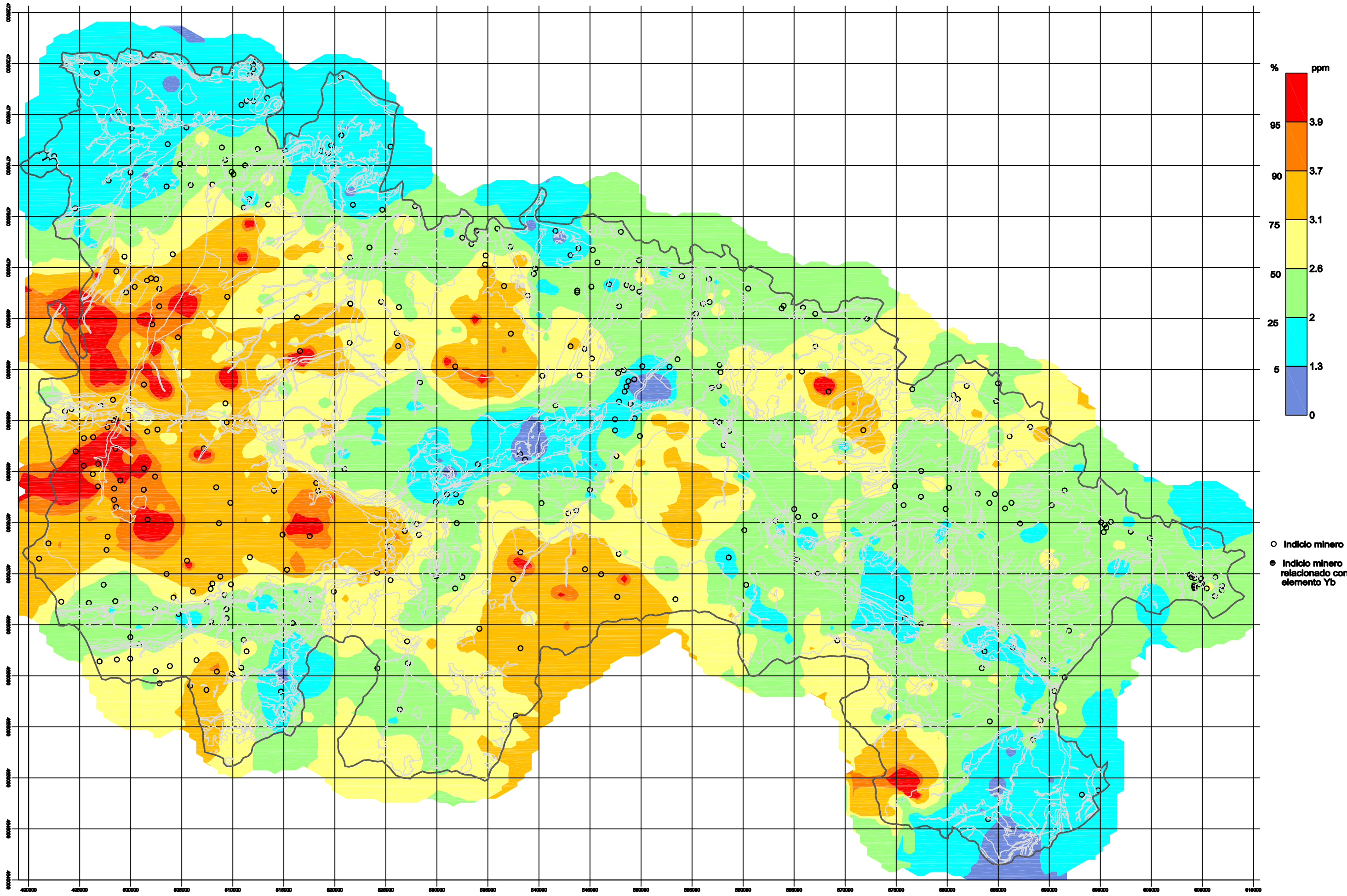
Figura 6.44: Tratamiento geoquímico univariante. Distribución del Yb
