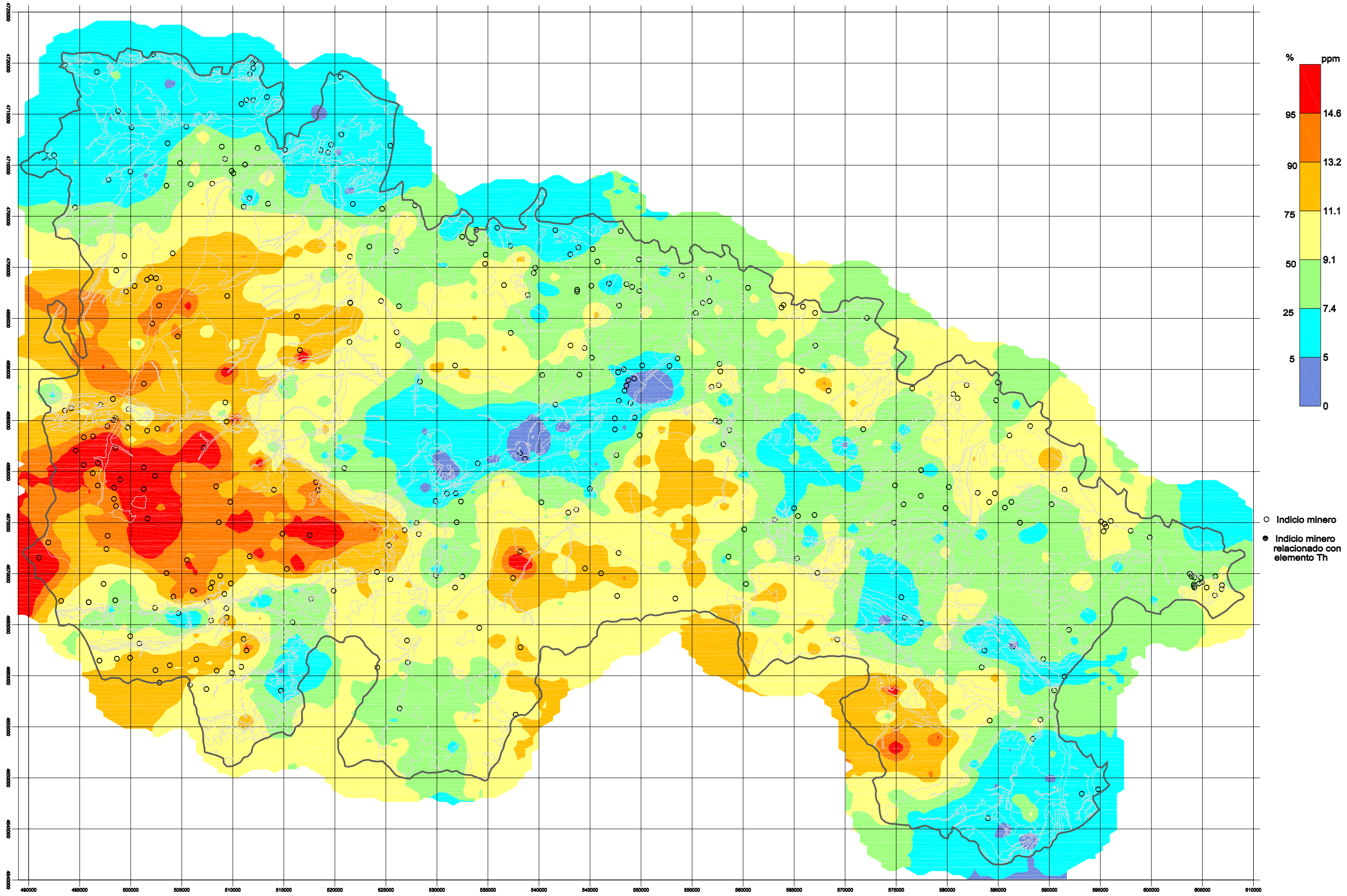
Figura 6.38: Tratamiento geoquímico univariante. Distribución del Th
