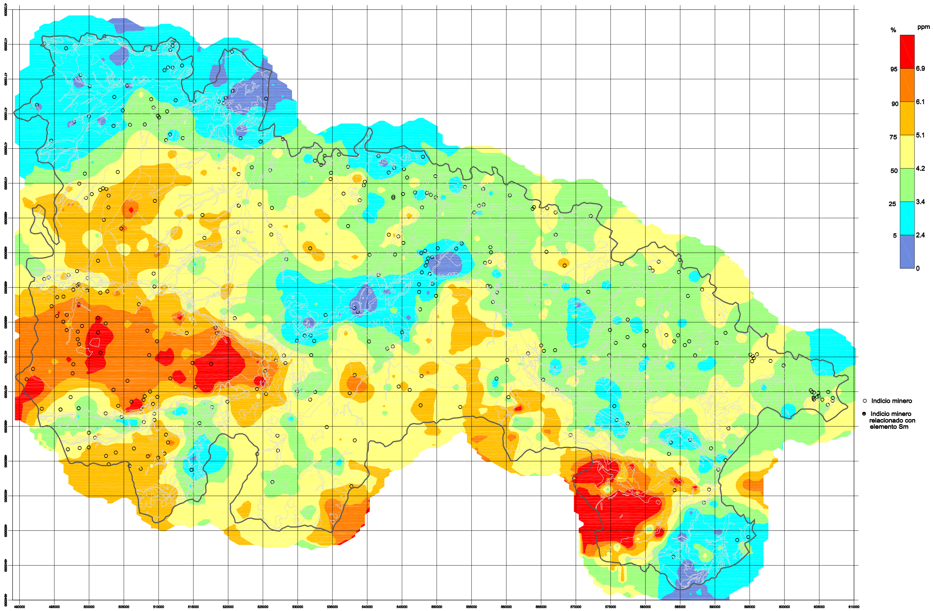
Figura 6.34: Tratamiento geoquímico univariante. Distribución del Sm
