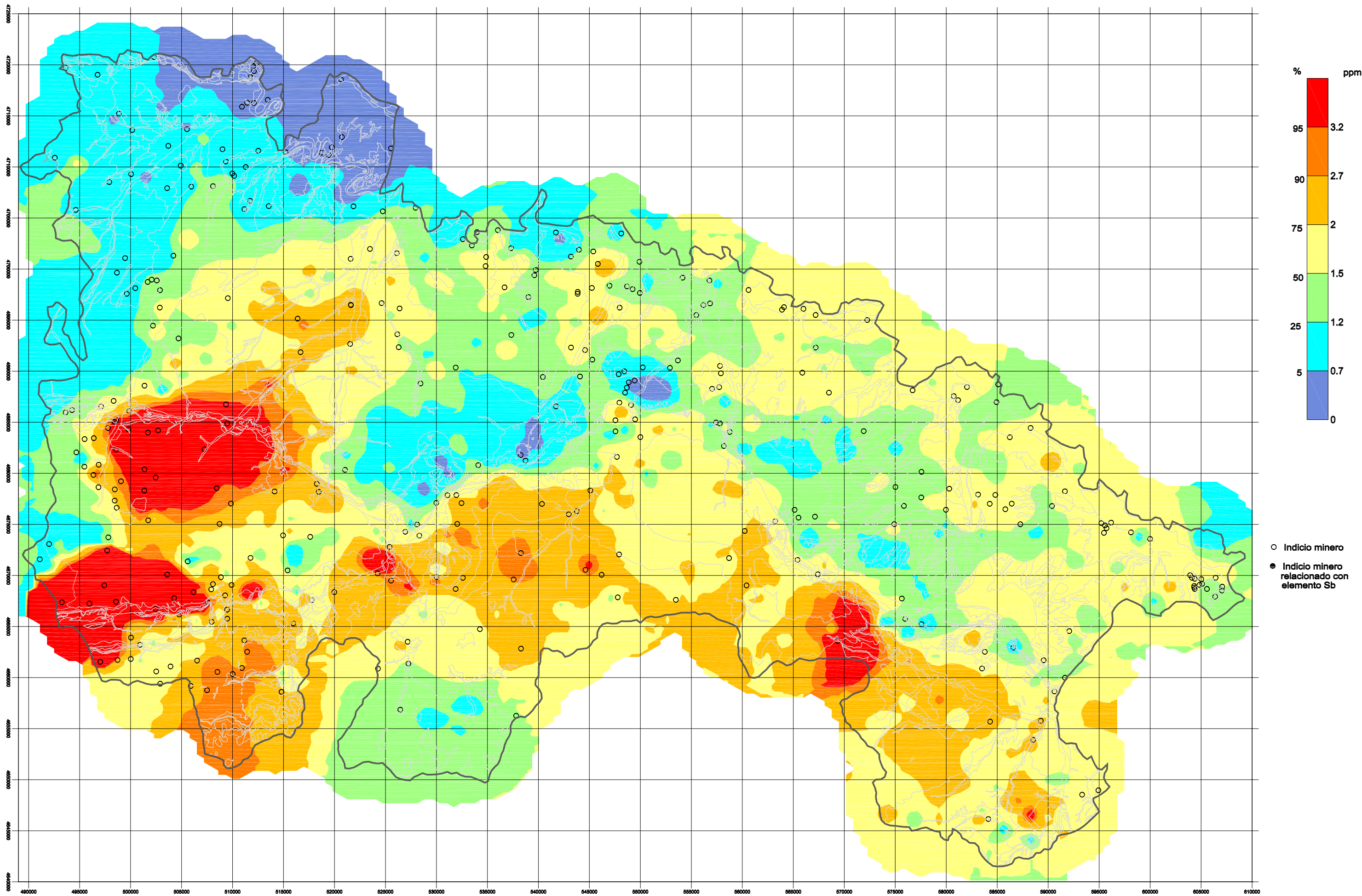
Figura 6.32 Tratamiento geoquímico univariante. Distribución del Sb
