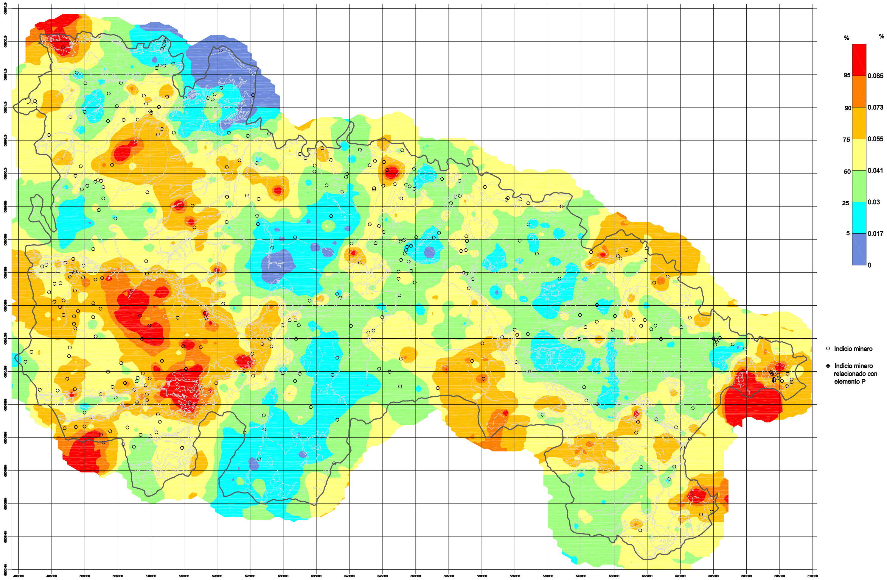
Figura 6.28: Tratamiento geoquímico univariante. Distribución del P
