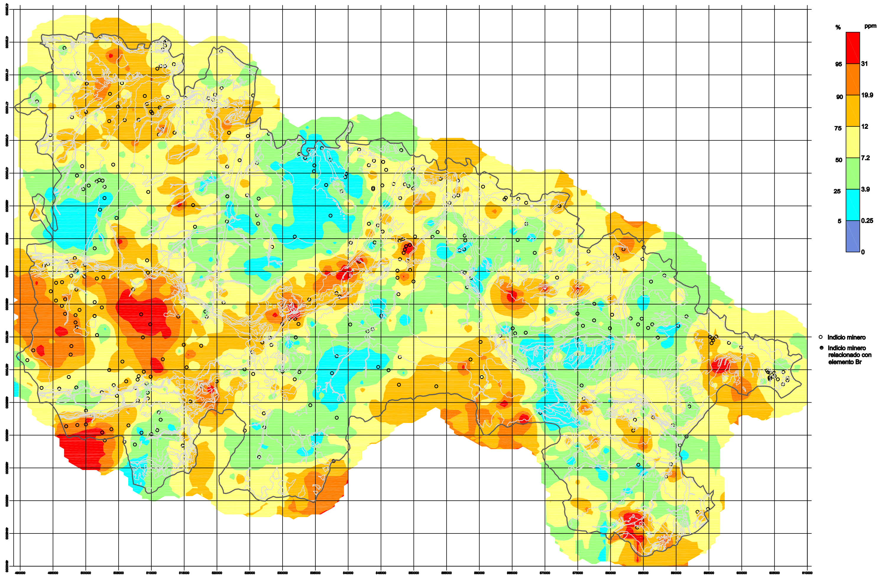
Figura 6.8: Tratamiento geoquímico univariante. Distribución del Br
