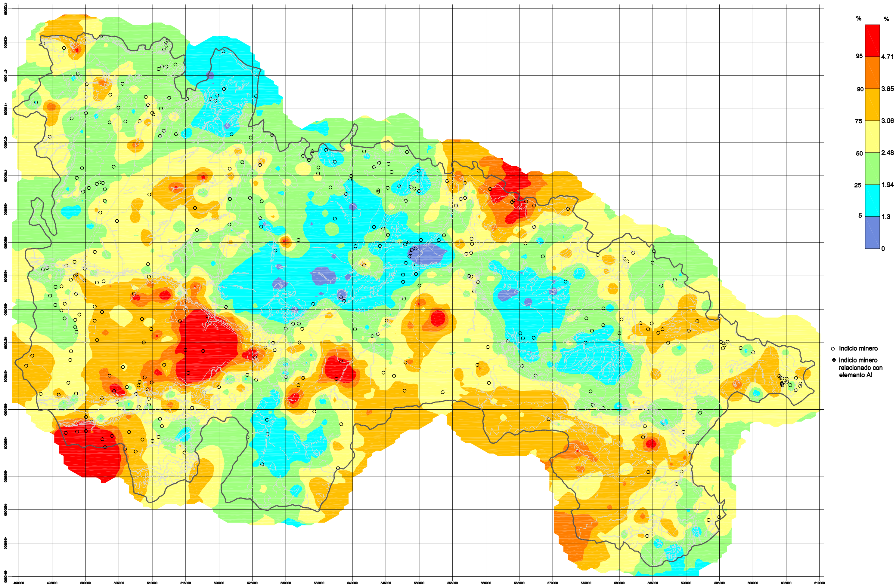
Figura 6.2: Tratamiento geoquímico univariante. Distribución del Al
