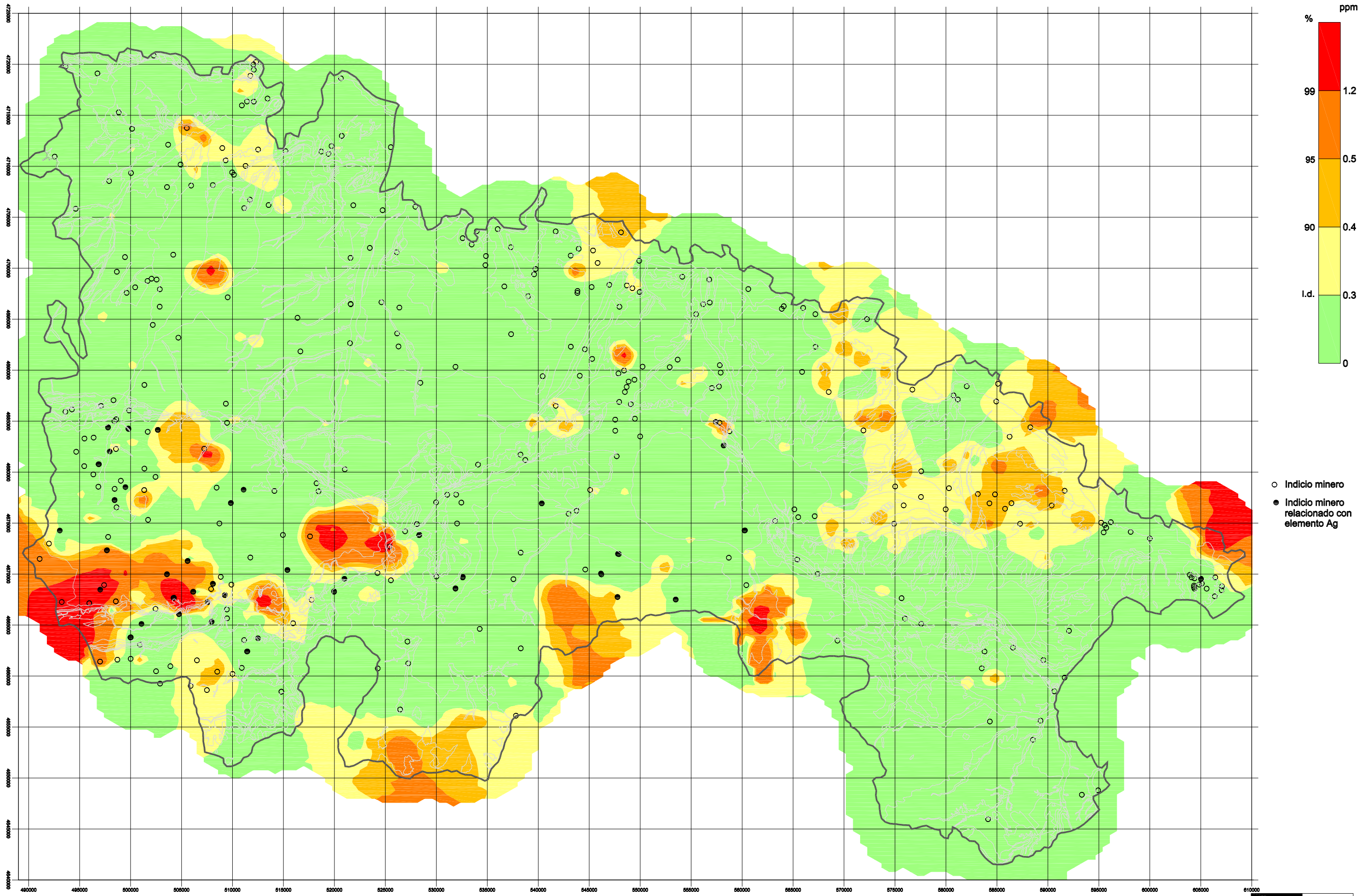
Figura 6.1: Tratamiento geoquímico univariante. Distribución de Ag
